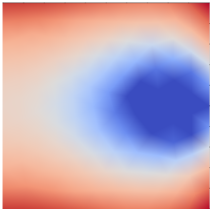
a) PI-GNN
