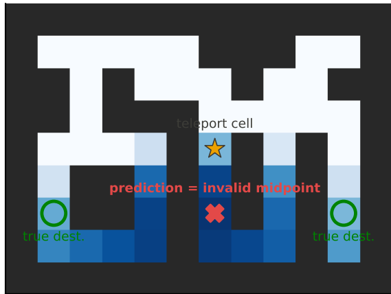
dense predictor (standard JEPA)
