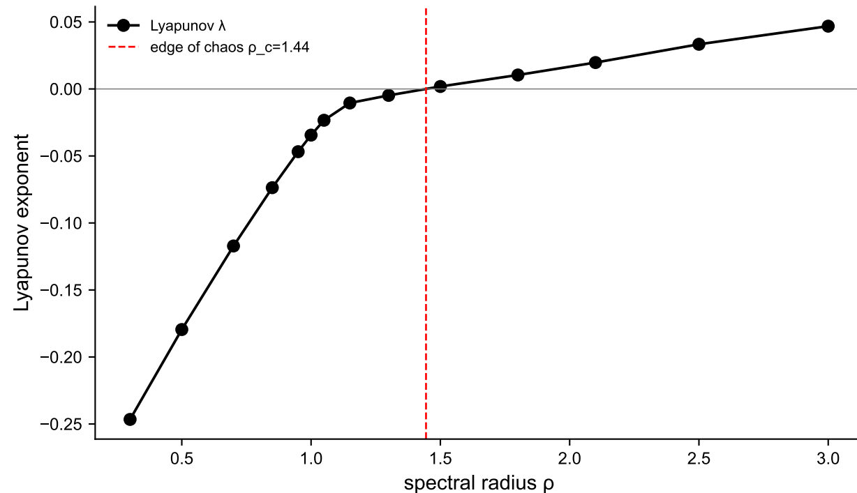
A. Locating the edge of chaos
