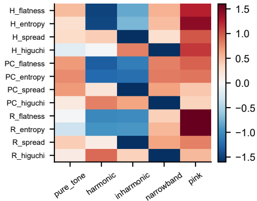
B Descriptor fingerprint (z per row)
