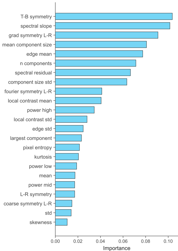
(a) Random Forest importance (Gini)
