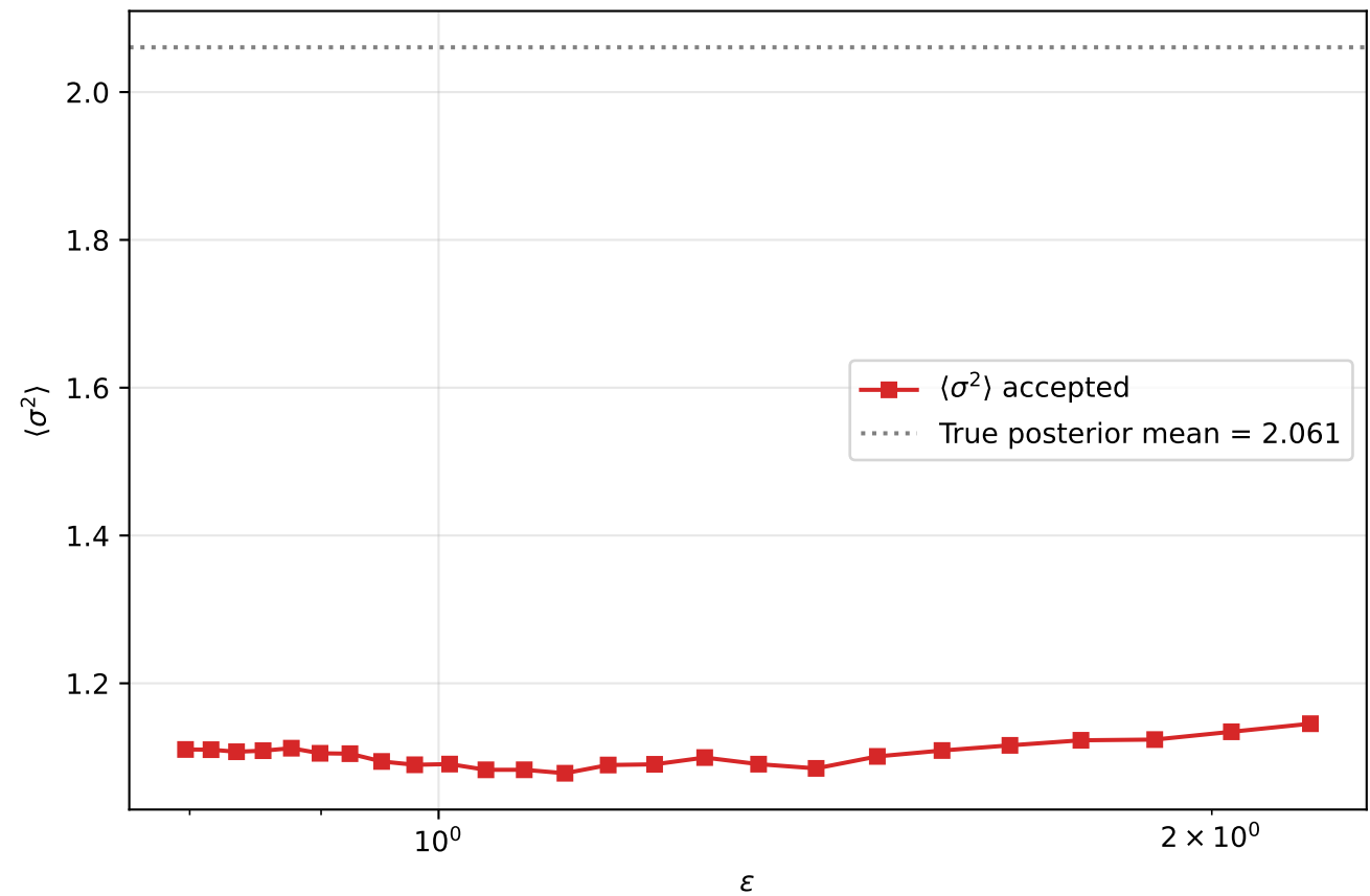
Posterior \sigma^2 bias vs \epsilon
