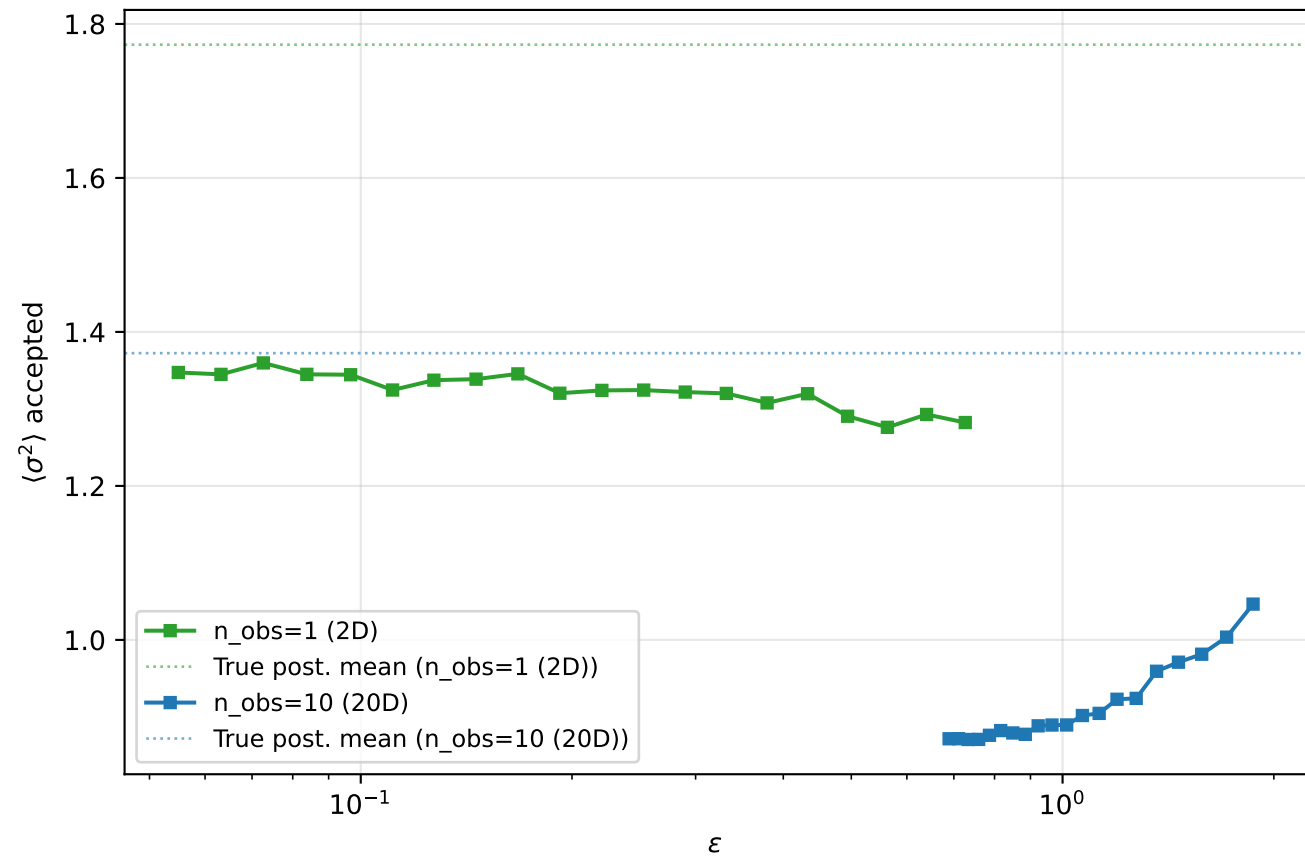
Posterior \sigma^2 bias vs \varepsilon
