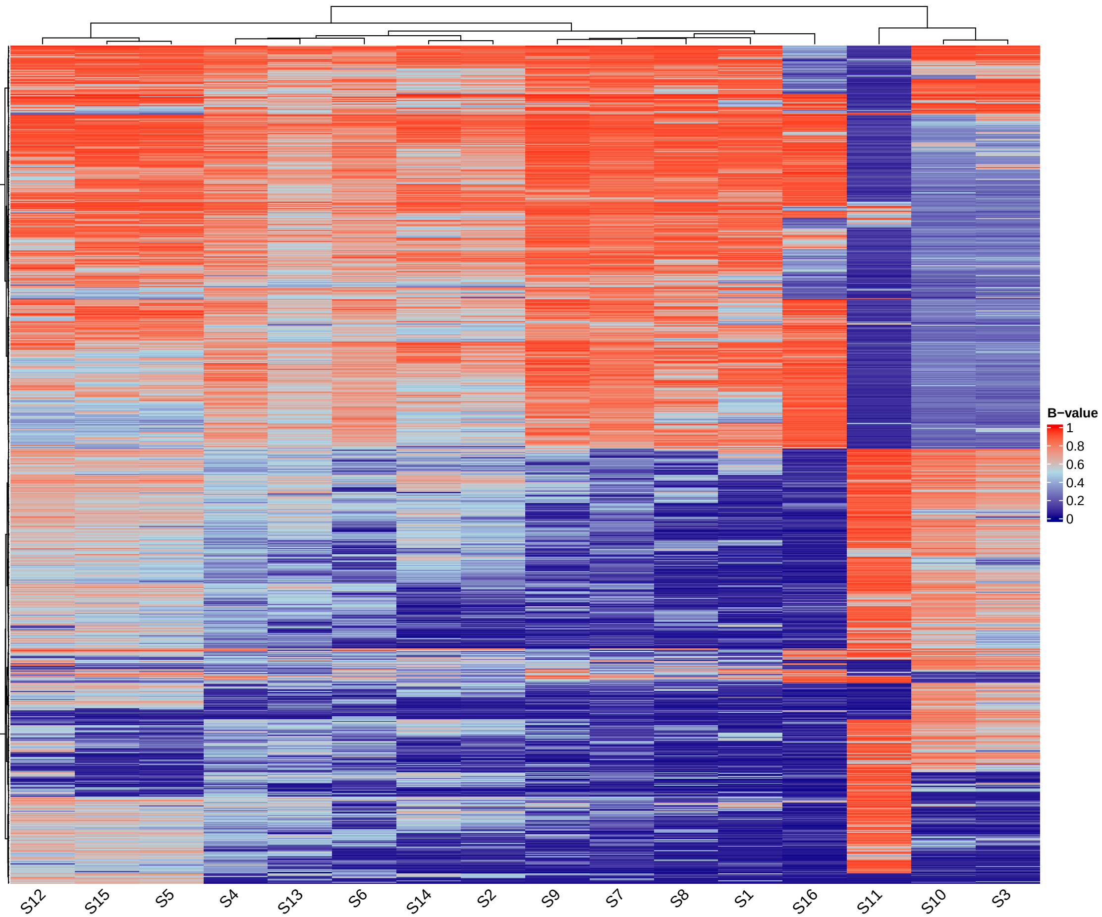
Profil de méthylation des lymphomes (1000 CpG les plus variables)
