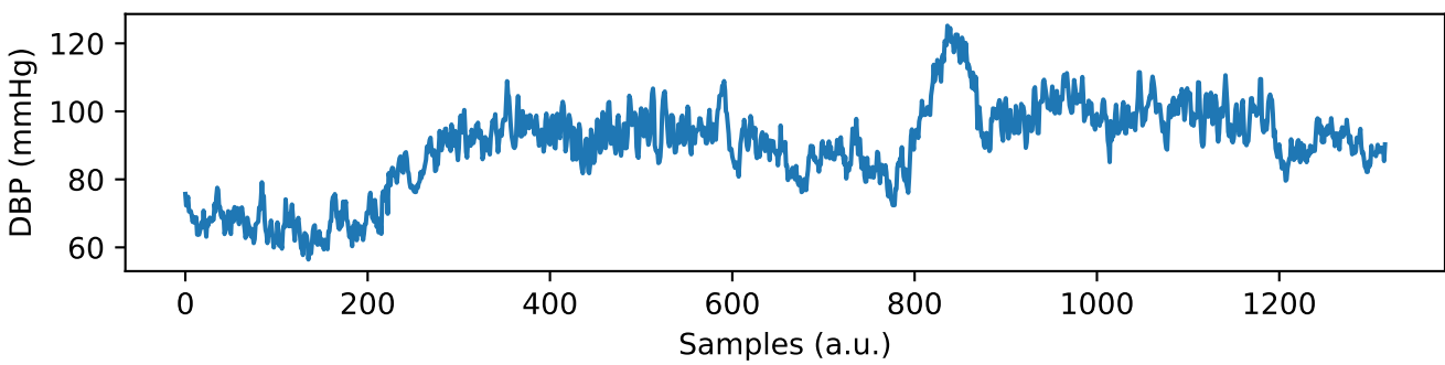
DBP
