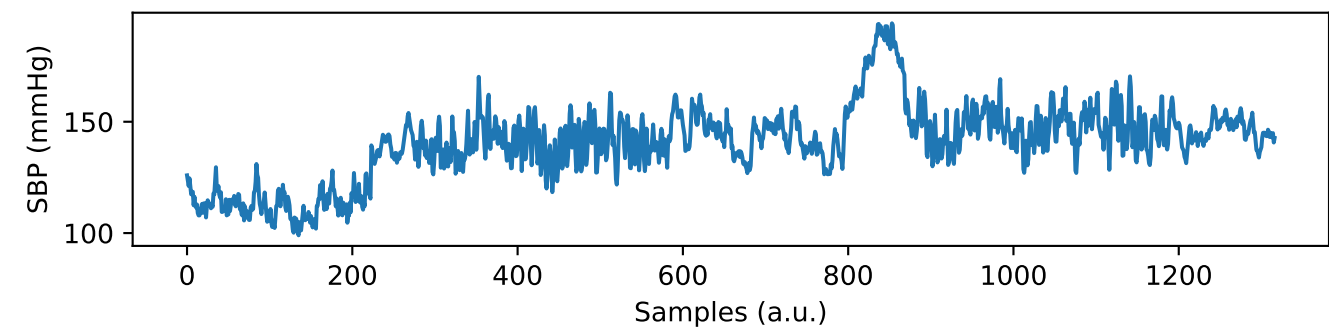
SBP
