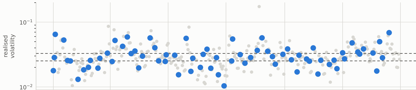
ETH/USDC
