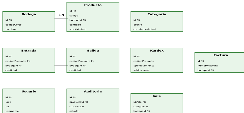
Diagrama Entidad-Relación (ERD) — Room Database v30
