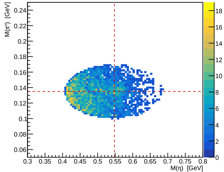
solo chi2
