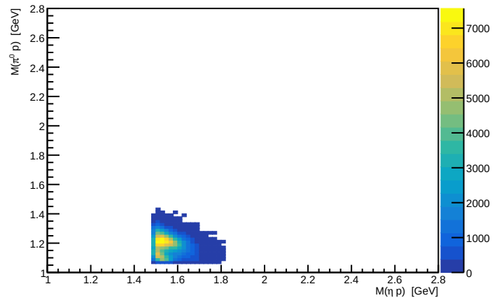
gate BDT - protone implicito
