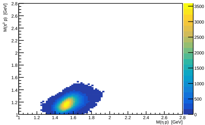
solo chi2 - protone implicito
