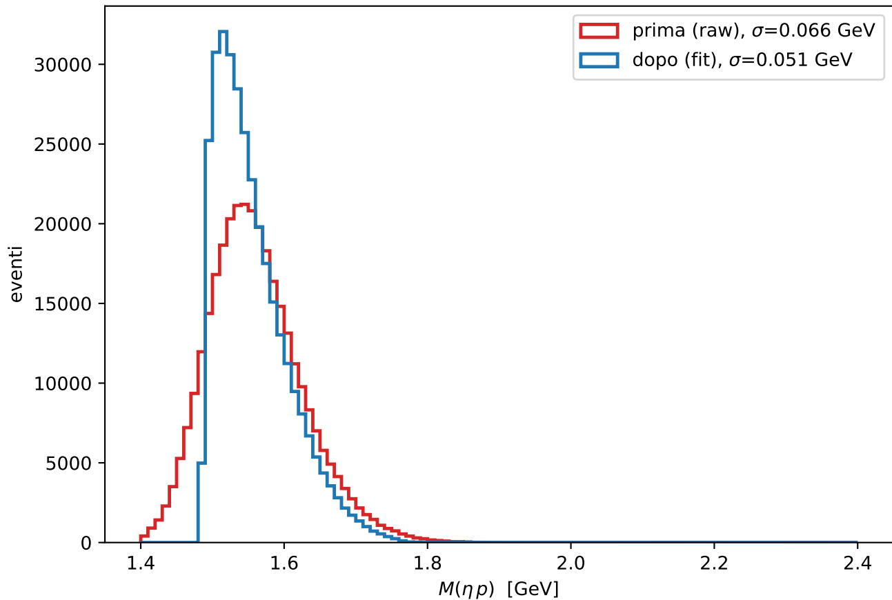
M(\eta p) : prima vs dopo il fit (dati, gate BDT)
