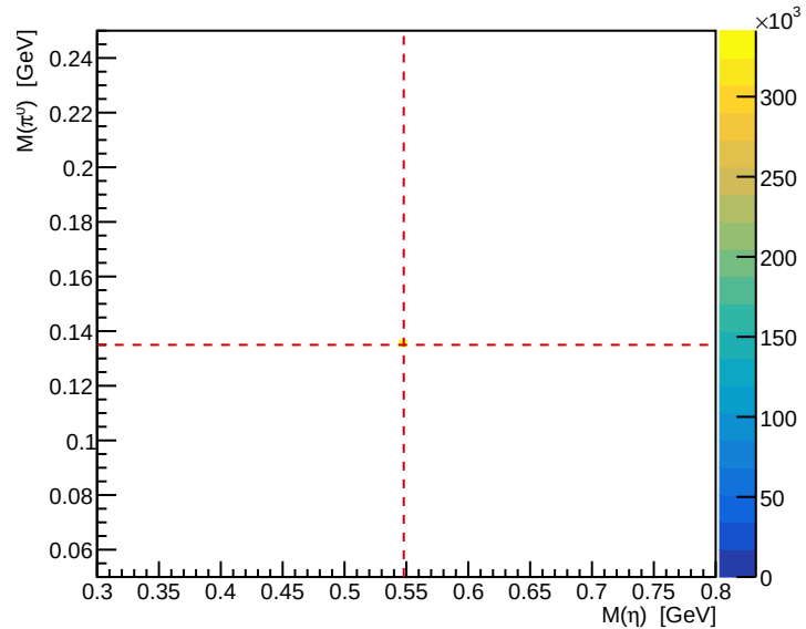
solo chi2
