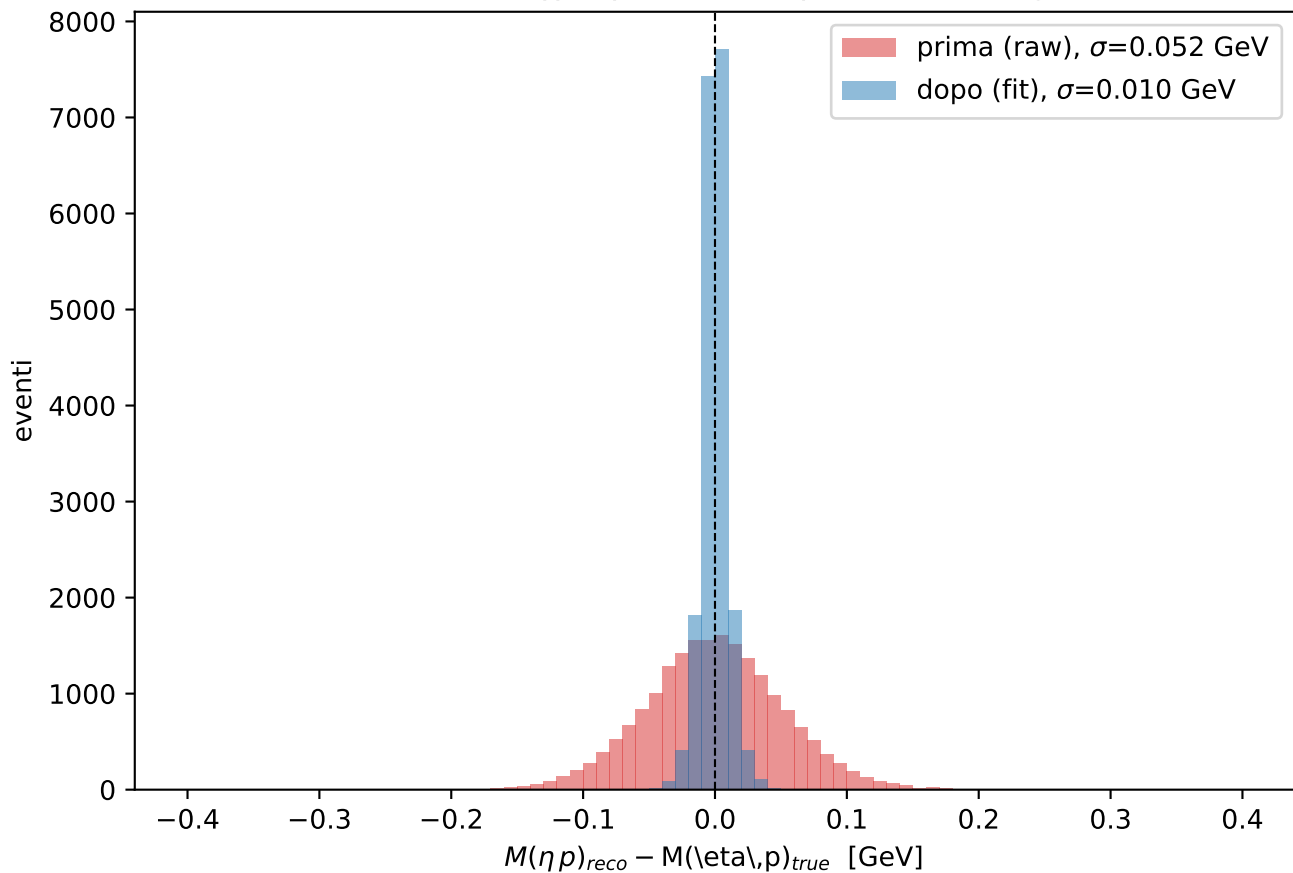
Risoluzione M(\eta p) : prima vs dopo il fit (MC segnale)
