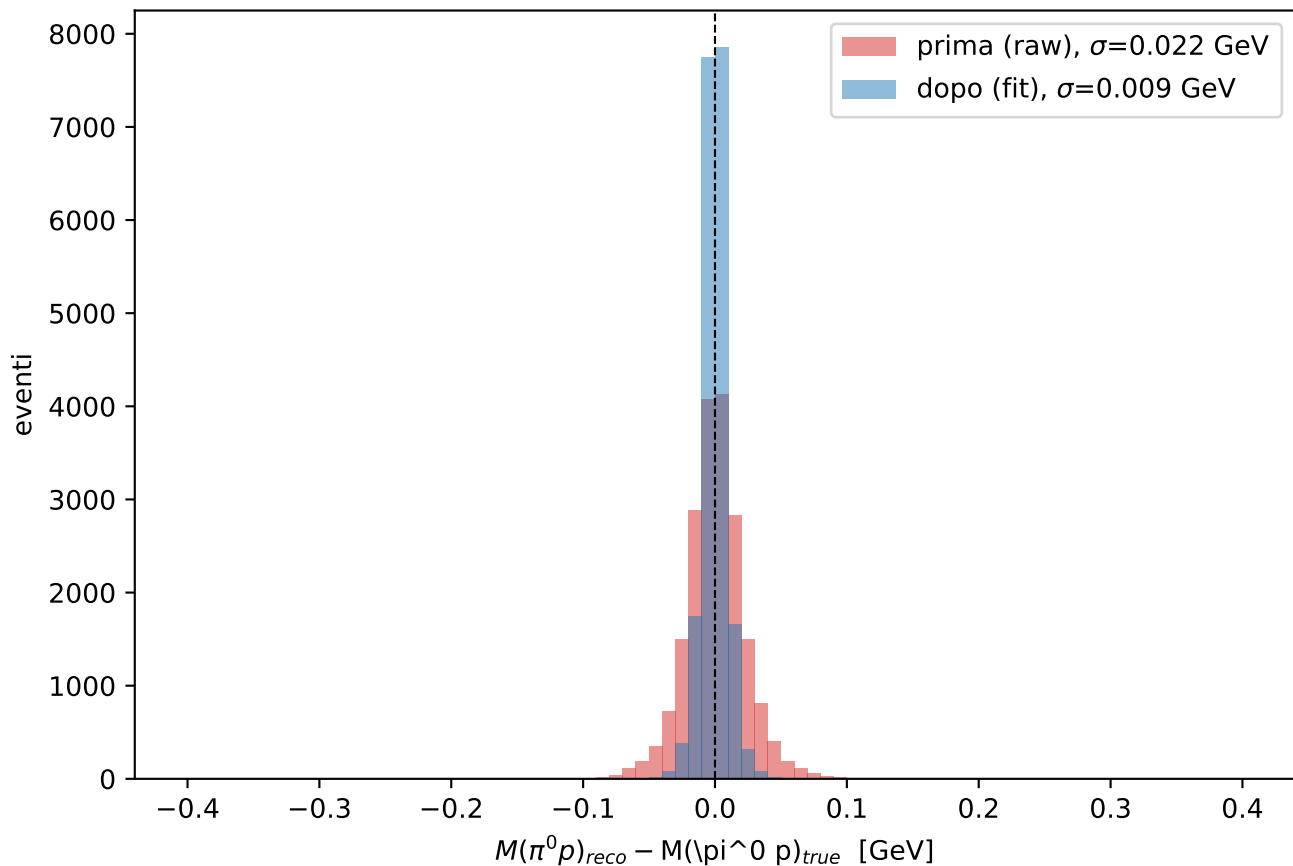
Risoluzione M(\pi^0 p) : prima vs dopo il fit (MC segnale)
