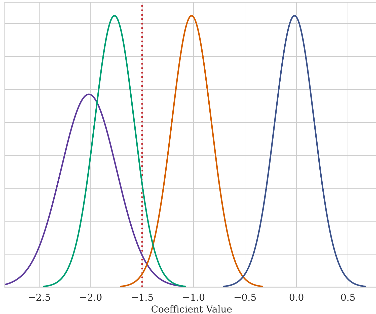
Posterior Density for \beta_3
