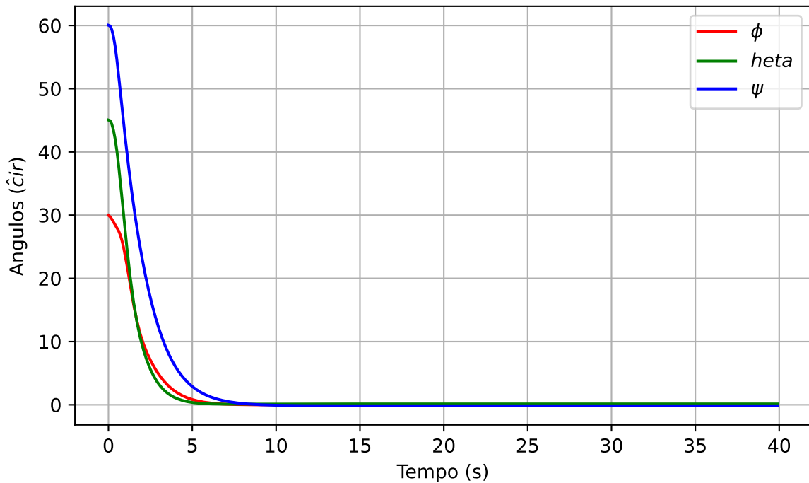
Ângulos de Euler do satélite
