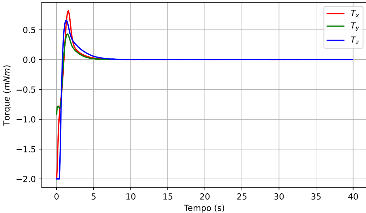
Torque de controle
