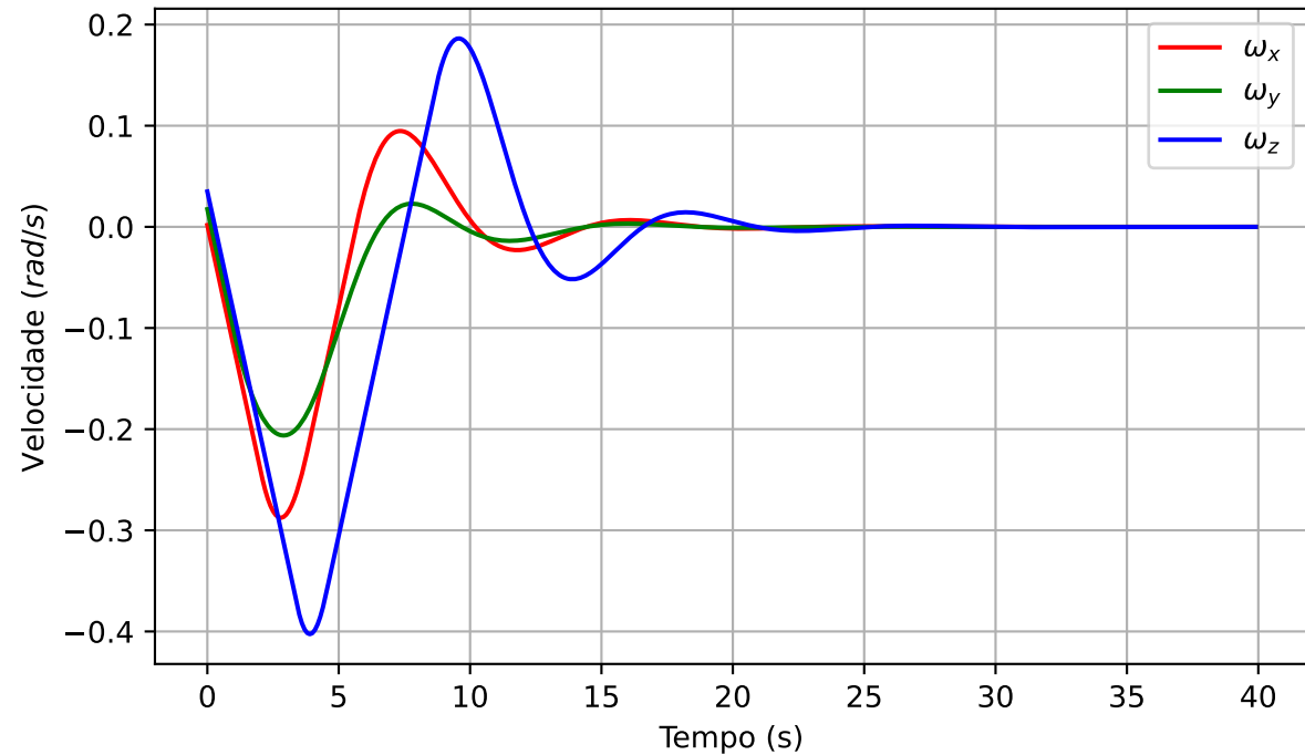
Velocidades angulares do satélite
