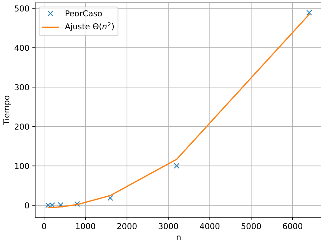
Peor caso \sim \Theta(n^2)
