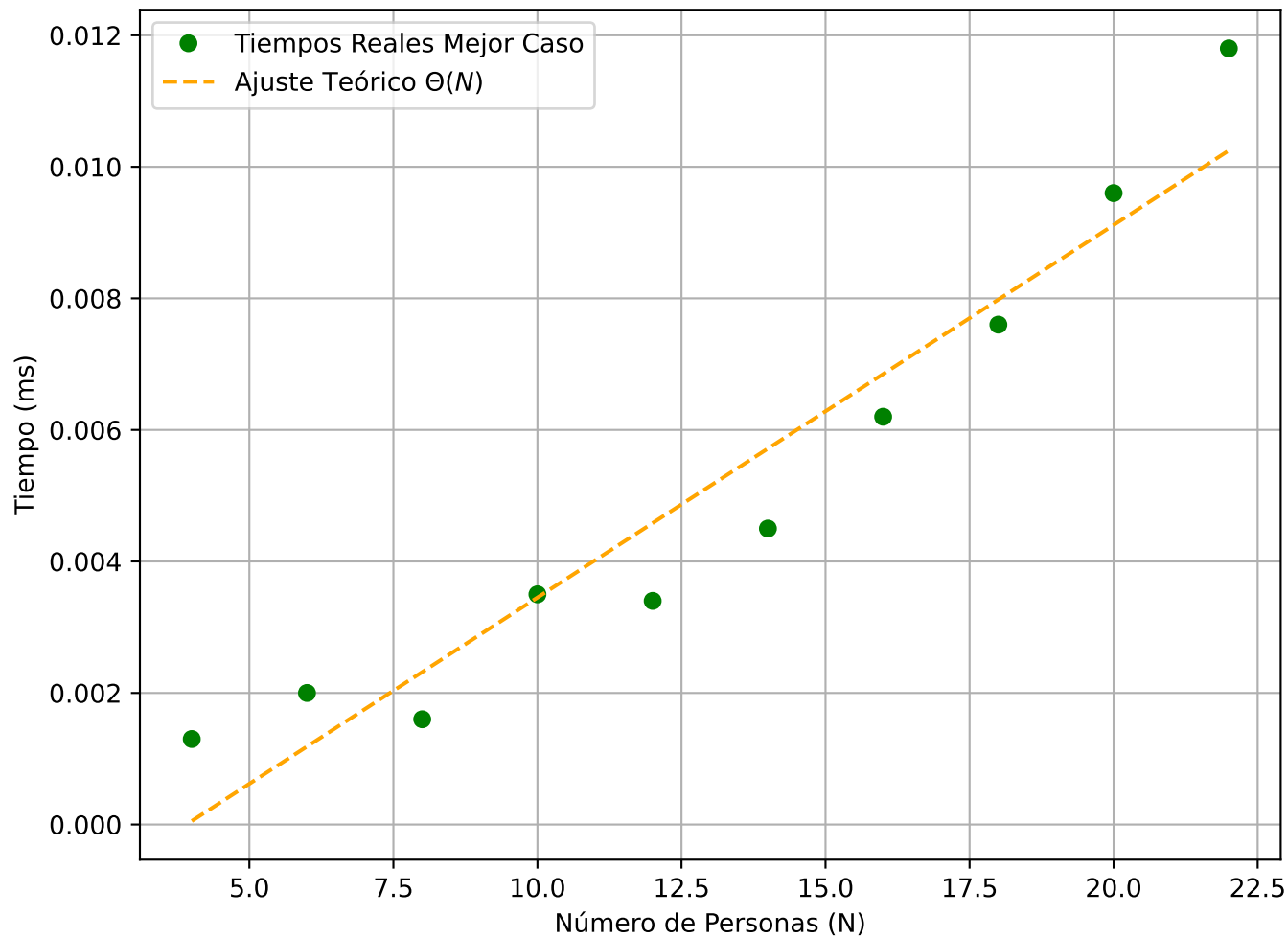
Contraste Teórico-Experimental Mejor Caso \sim \Theta(N)
