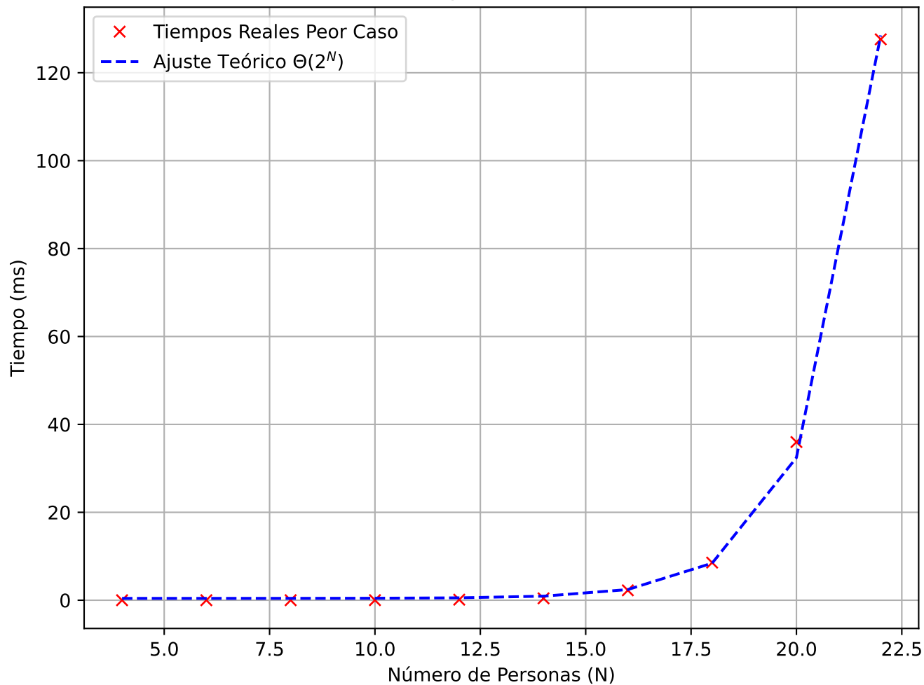
Contraste Teórico-Experimental Peor Caso \sim \Theta(2^N)
