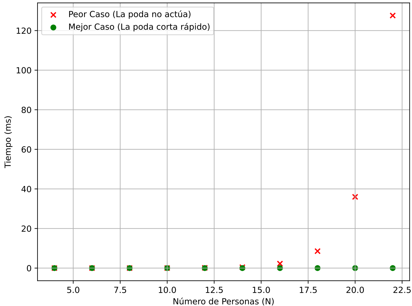
Comparativa de Tiempos: Efecto de la Poda en Backtracking
