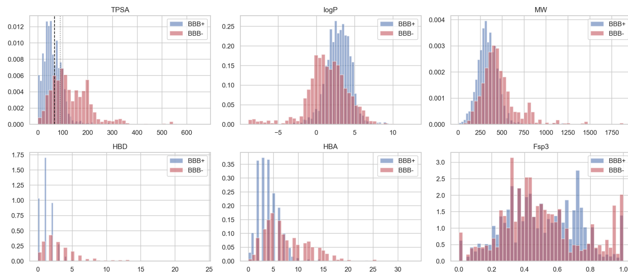
Figura 2: Distribución de TPSA, logP, MW, HBD, HBA y Fsp3, separada por clase. Las líneas verticales en TPSA marcan los umbrales de 66.8 y 90 Å² reportados en la literatura.
