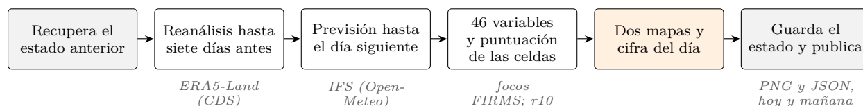
Figura 8: Pasos de la cadena diaria en GitHub Actions. En cursiva, la fuente o el producto de cada paso. CDS es el Climate Data Store de Copernicus.
