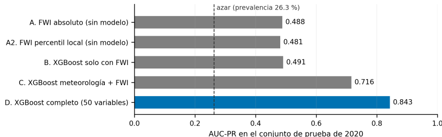
Figura 5: AUC-PR en el conjunto de prueba de 2020 de cada peldaño de la primera iteración, del FWI sin modelo al XGBoost con 50 variables. La línea discontinua marca el azar, que en esta métrica coincide con la proporción de positivos.
