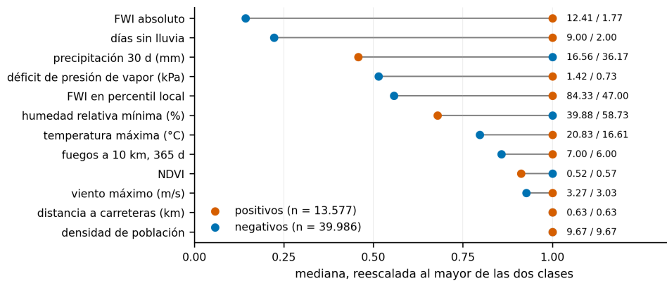
Figura 4: Medianas de positivos y negativos en el conjunto de entrenamiento de la primera iteración (2015–2018). Las variables meteorológicas separan los dos grupos; las del territorio coinciden.
