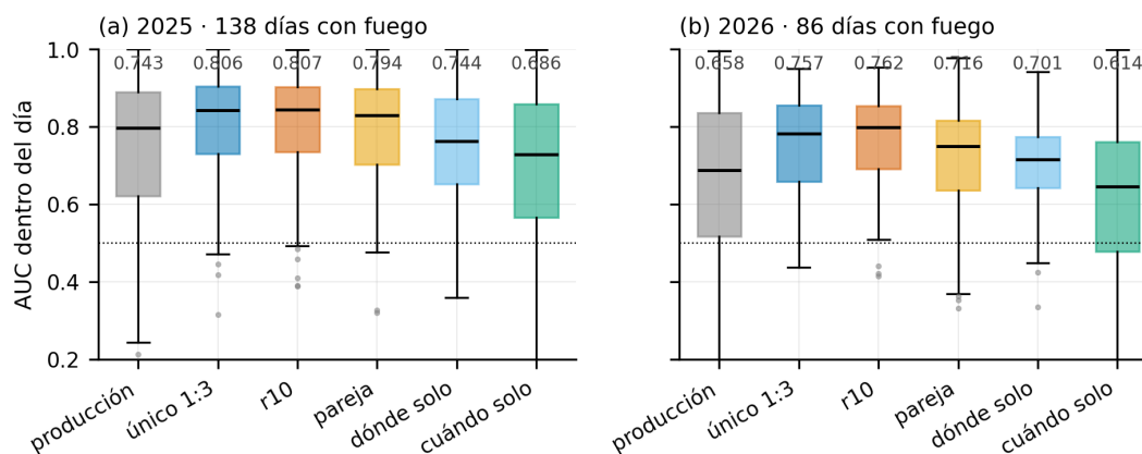
Figura 7: AUC dentro del día de los seis modelos en los días con fuego de cada temporada, con la previsión de la víspera. Caja: cuartiles y mediana; bigotes: 1.5 veces el rango intercuartílico. La cifra sobre cada caja es la media de la tabla 6; la línea de puntos, el azar.
