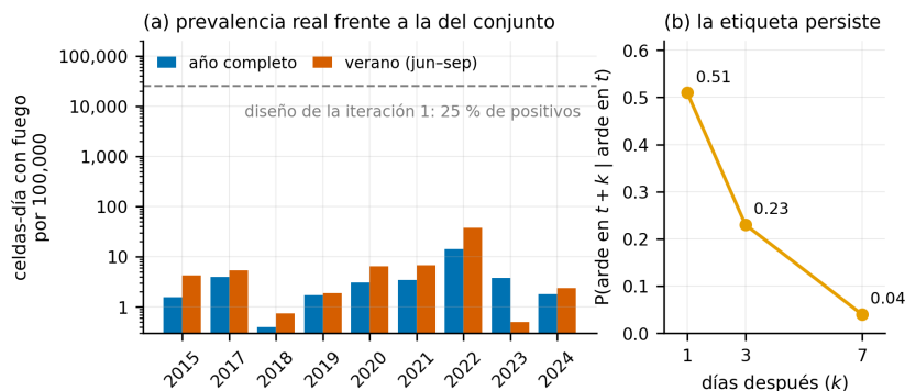
Figura 2: (a) Celdas-día con fuego por cada 100,000 según EFFIS, año completo y verano, en escala logarítmica, frente a la proporción de positivos del primer diseño. (b) Probabilidad de que una celda siga marcada como quemada k días después.
