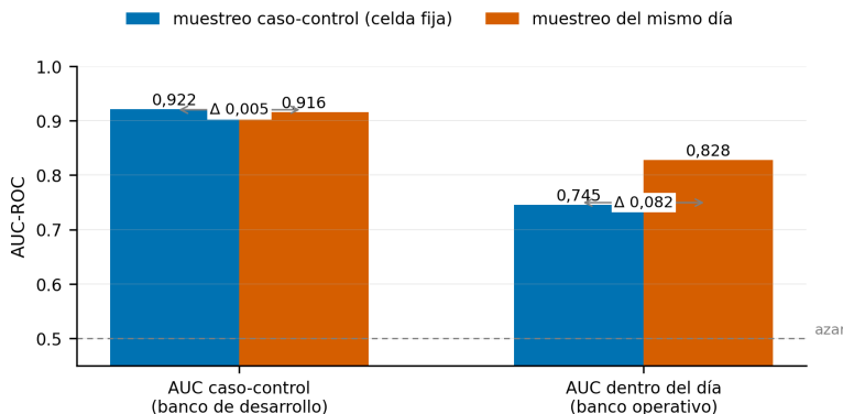
Figura 6: Los dos diseños de muestreo bajo dos métricas. El AUC caso-control, medido con el conjunto de prueba de cada diseño, es igual para los dos; el AUC dentro del día, en el conjunto de prueba de 2020, los separa.
