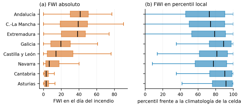
Figura 3: FWI en los días de incendio del periodo de entrenamiento, por comunidad autónoma. (a) Valor absoluto. (b) Percentil respecto a la historia de la propia celda.
