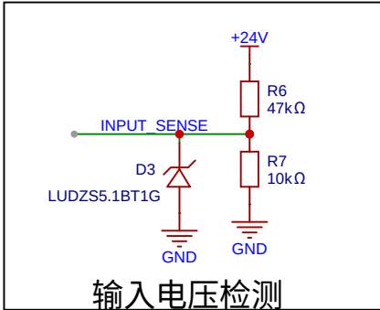
24V输入
