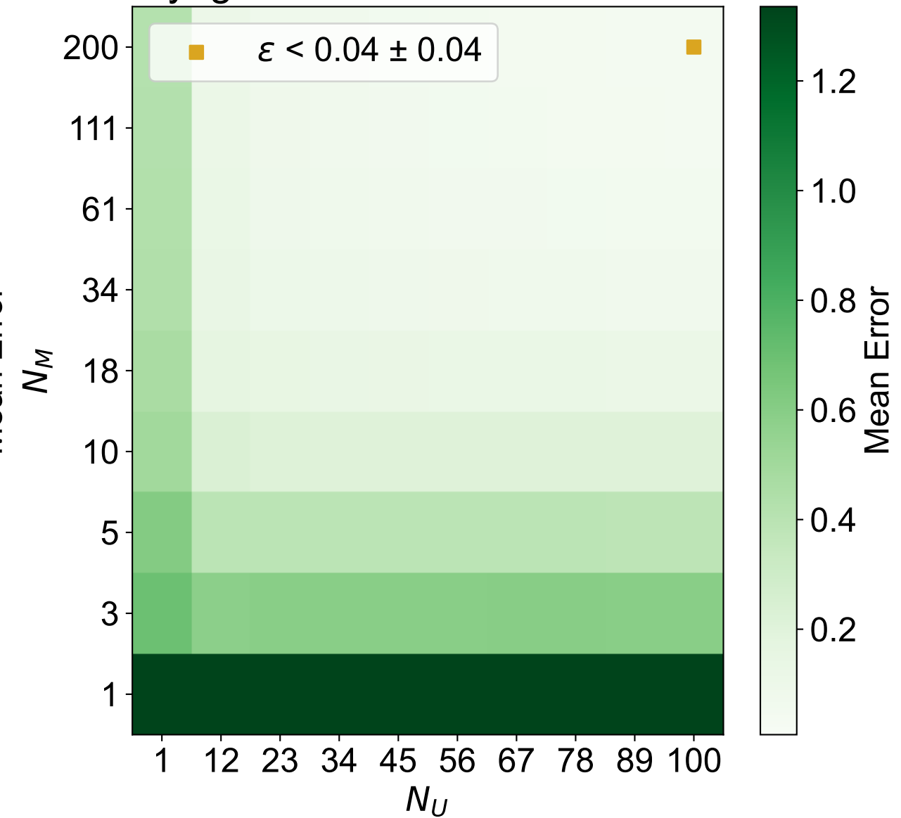
Brydges et al Mean Error Surface
