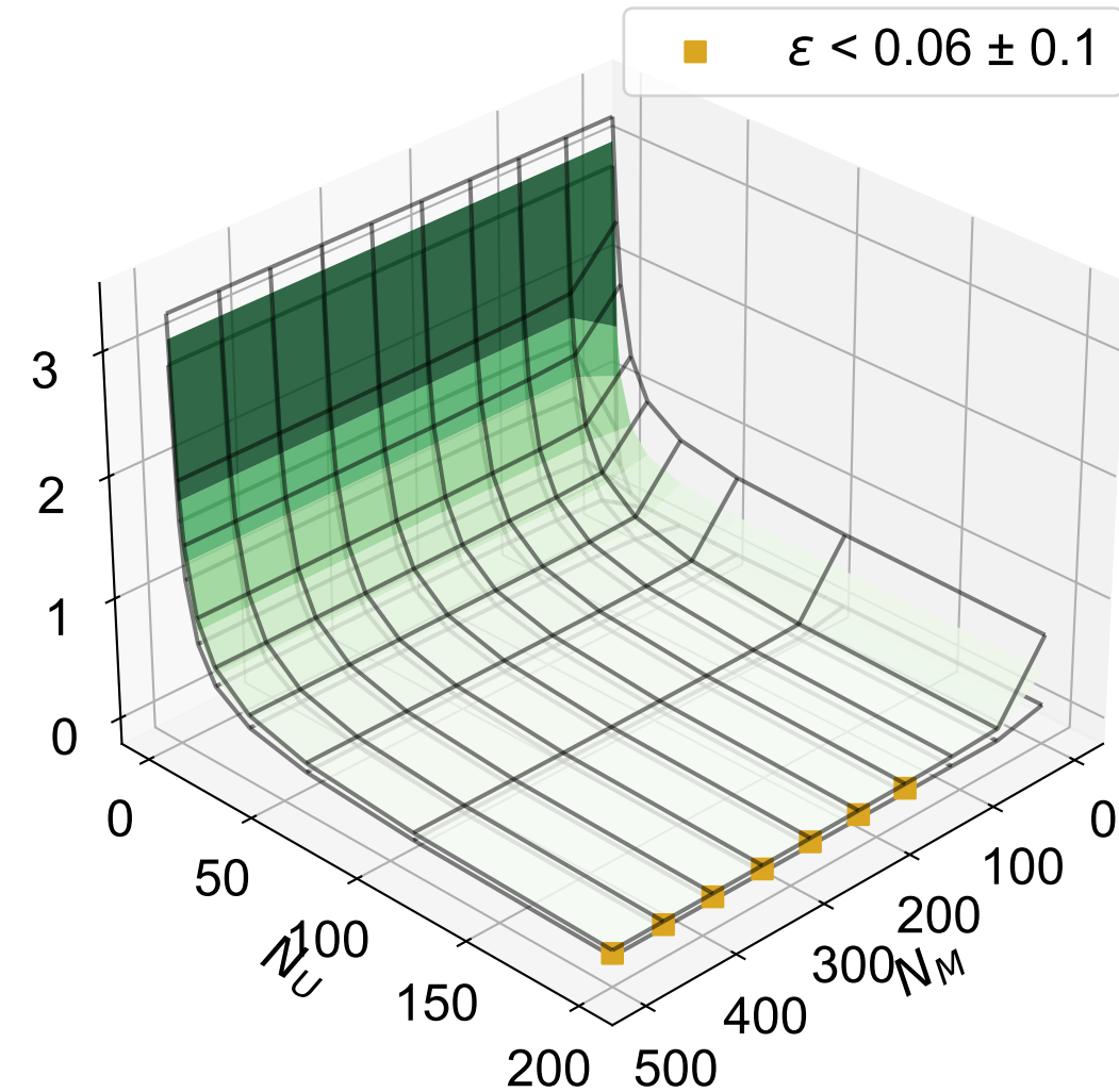
Brydges et al Mean Error Surface
