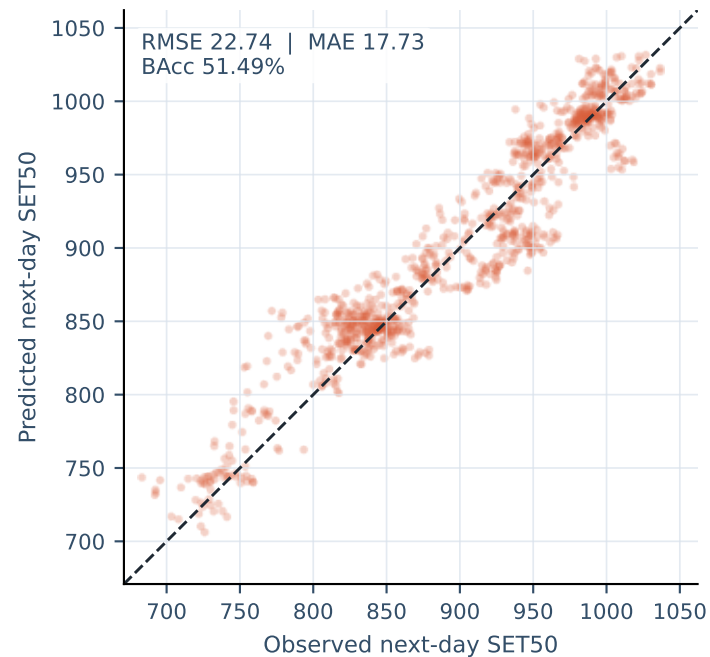
CNN
