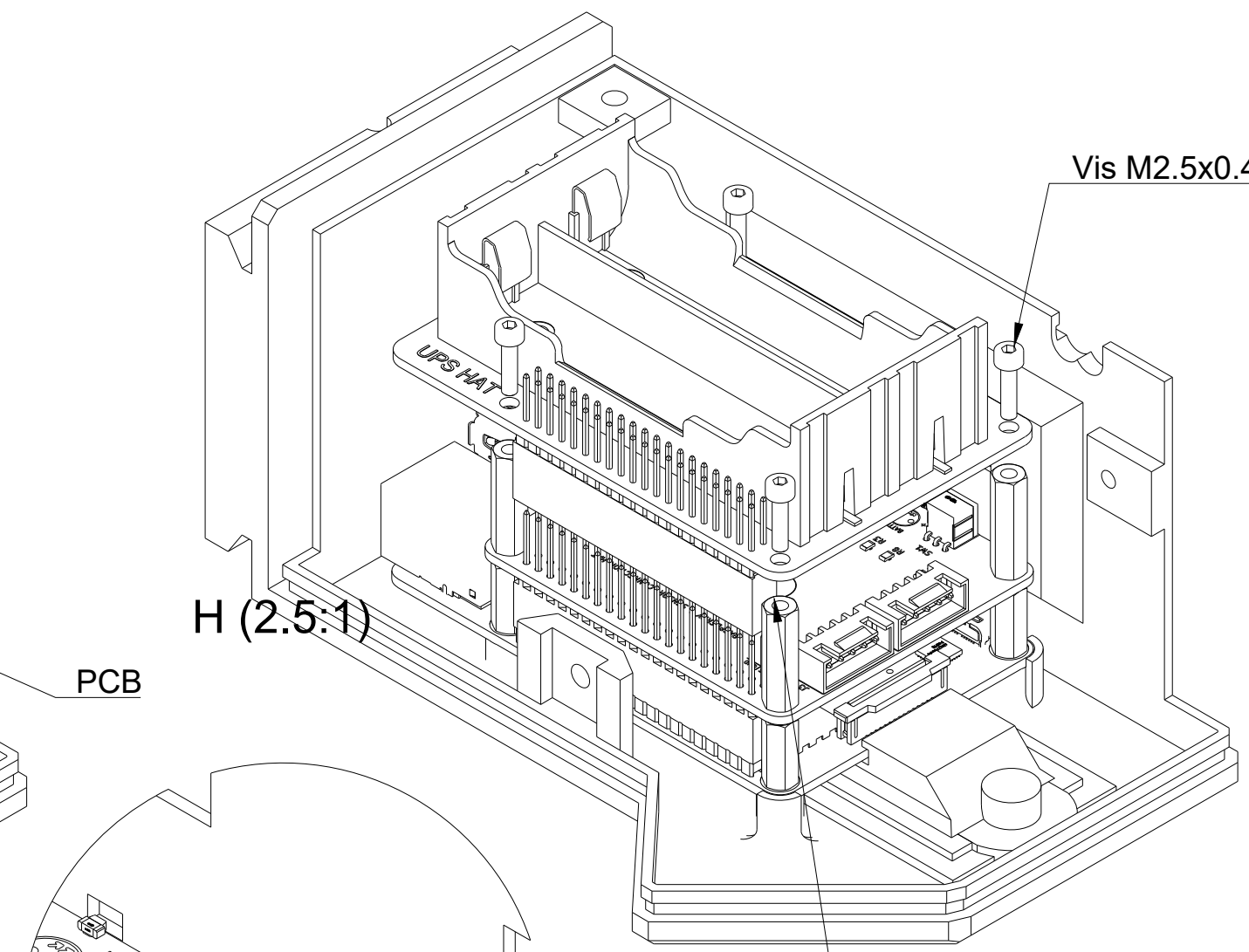
15 : Branchement du PCB d'alimentation
