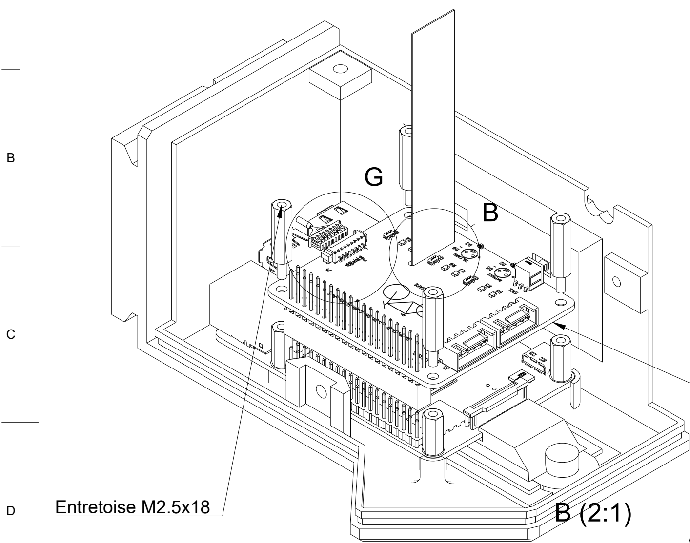
14: Branchement du PCB de connections pour les capteurs.
