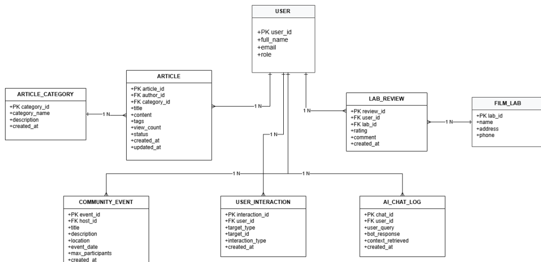
Hình 3.4: Sơ đồ quan niệm ERD phân hệ Knowledge & AI Integration
