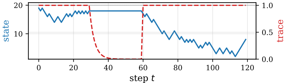
\lambda = 0.7 (ETTA)
