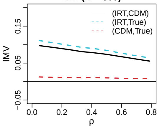
IMV (N = 500)
