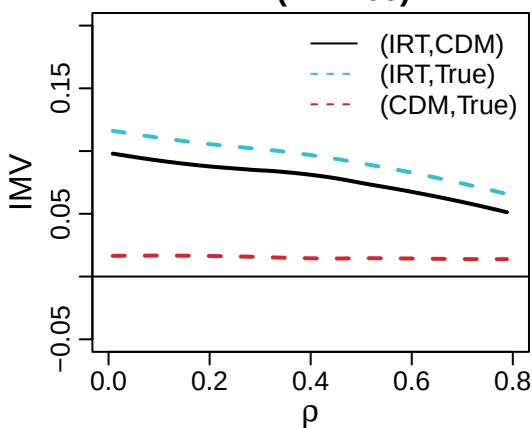
IMV (N = 200)
