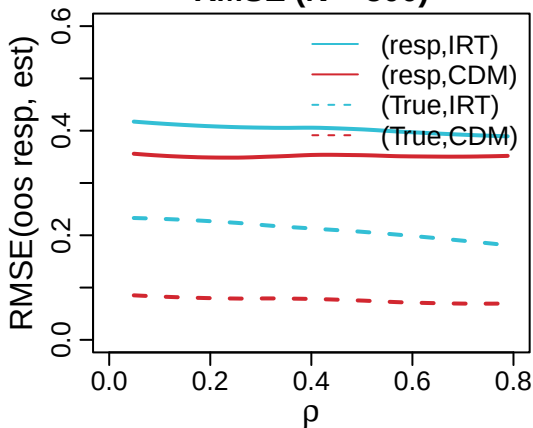
RMSE (N = 500)
