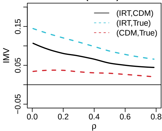
IMV (N = 500)
