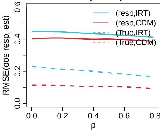
RMSE (N = 500)
