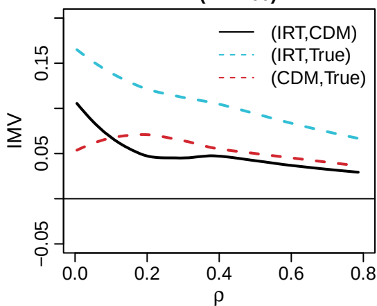
IMV (N = 200)
