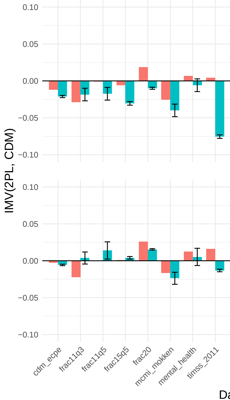
DINA
