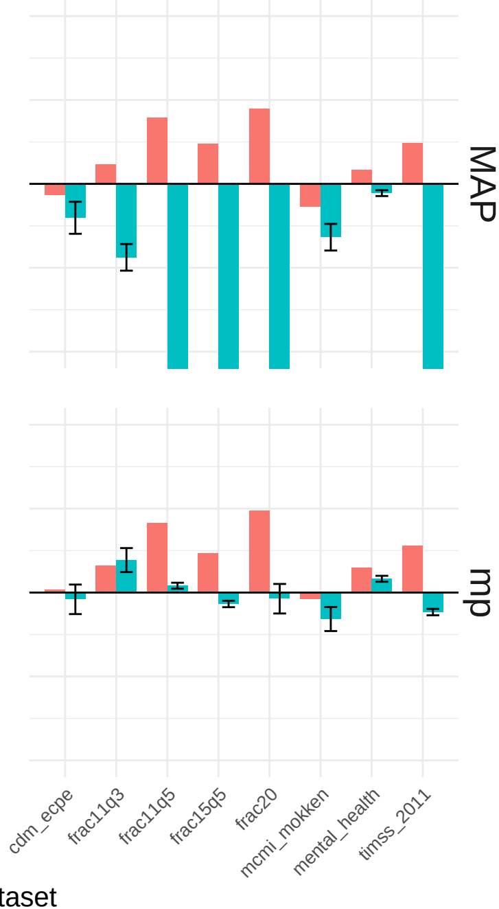
GDINA
