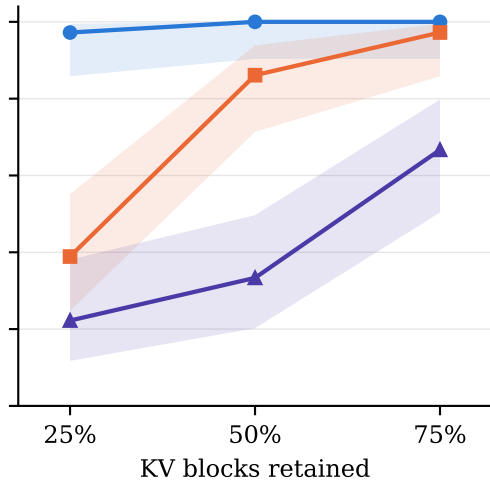
Qwen3-8B
