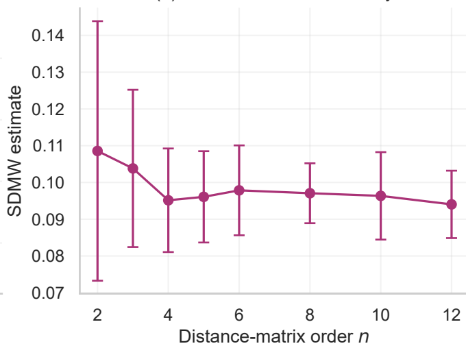
(d) Estimates with uncertainty
