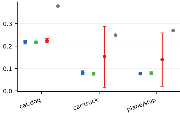
ViT-B/16
