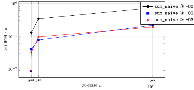
图 4.5: 求和题中 sum_naive 在不同优化等级下的运行时间
