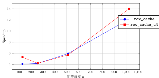
图 4.1: -03 下矩阵题相对 col_naive 的加速比
