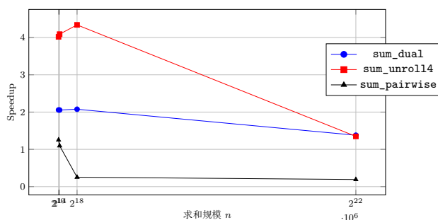
图 4.4: -03 下求和题相对 sum_naive 的加速比
