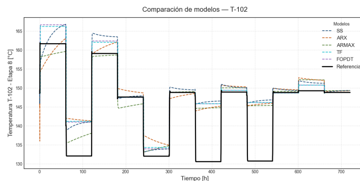
Figura 4. Comparación de los modelos subrogados respecto a los datos de validación para la columna T -102.
