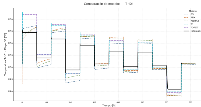
Figura 3. Comparación de los modelos subrogados respecto a los datos de validación para la columna T -101.
