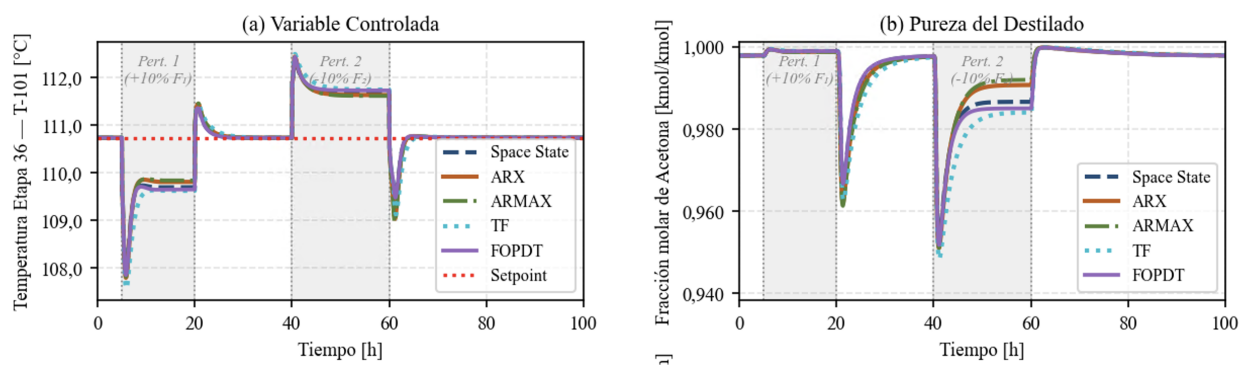
Figura 5. Evolución temporal de la variable controlada de T-101 bajo una perturbación del 10 % seguida de una perturbación del -10 %.
