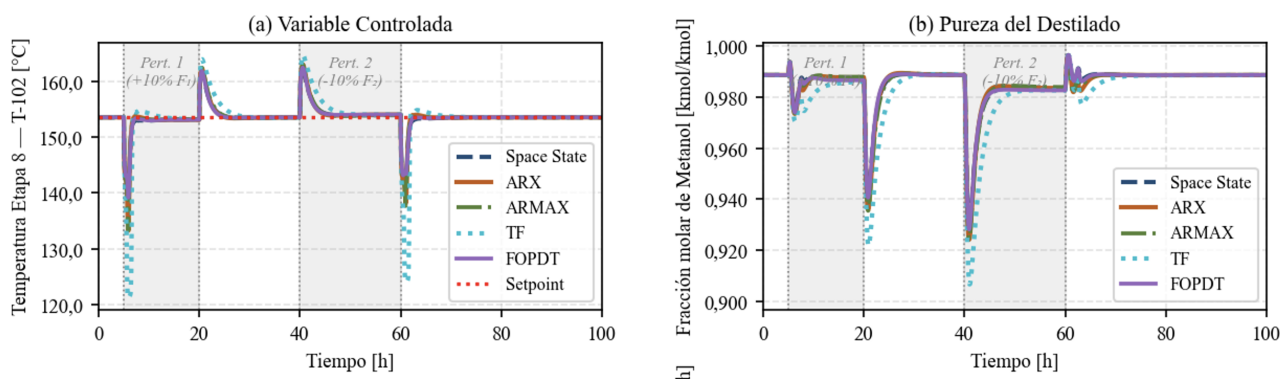
Figura 6. Evolución temporal de la variable controlada de T-102 bajo una perturbación del 10 % seguida de una perturbación del -10 %.
