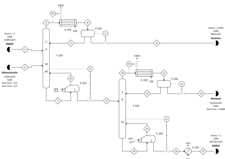
Figura 6. Diagrama del proceso de destilación extractiva.
