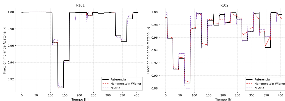
Figura 3. Comparación de los modelos subrogados del sistema para la columna T-101. y T-102.
