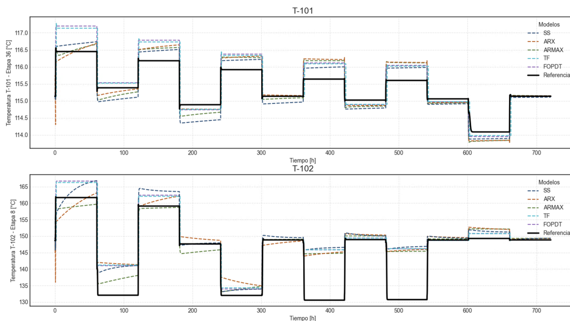
Figura 4. Comparación de los modelos subrogados respecto a los datos de validación para la columna T-101 y T-102.
