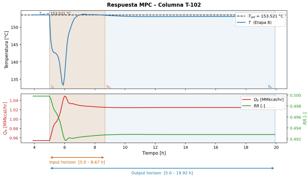
Figura 2. Ejemplo MISO de la esquematica de un controlador MPC utilizando la T-102.
