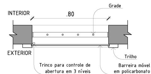
PLANTA ESCALA 1:25
