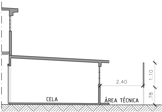
CORTE ESC: 1/100
