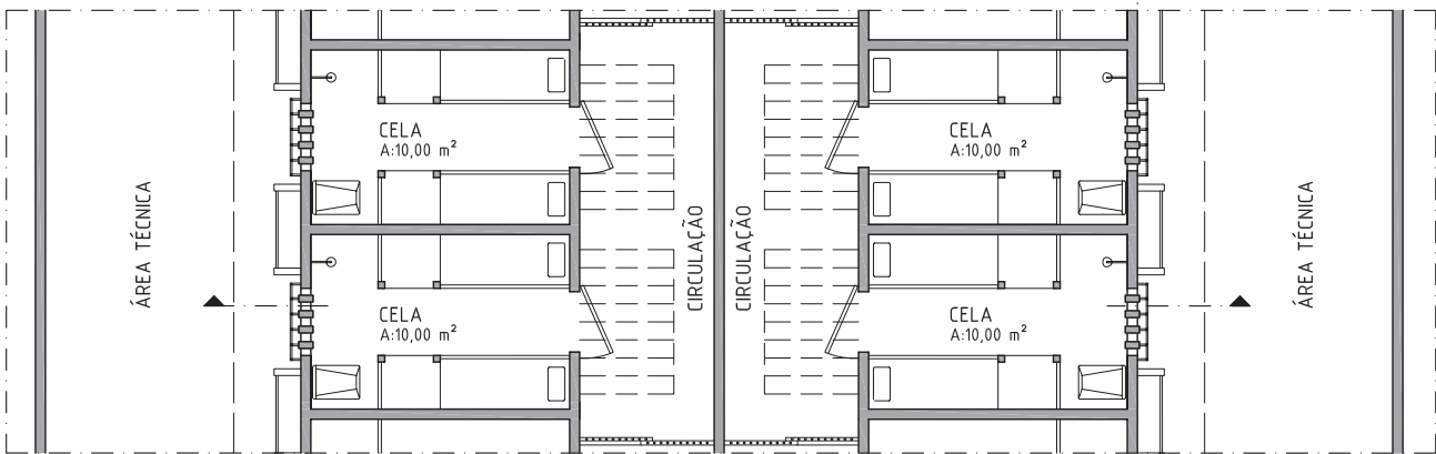
PLANTA ESC: 1/125
