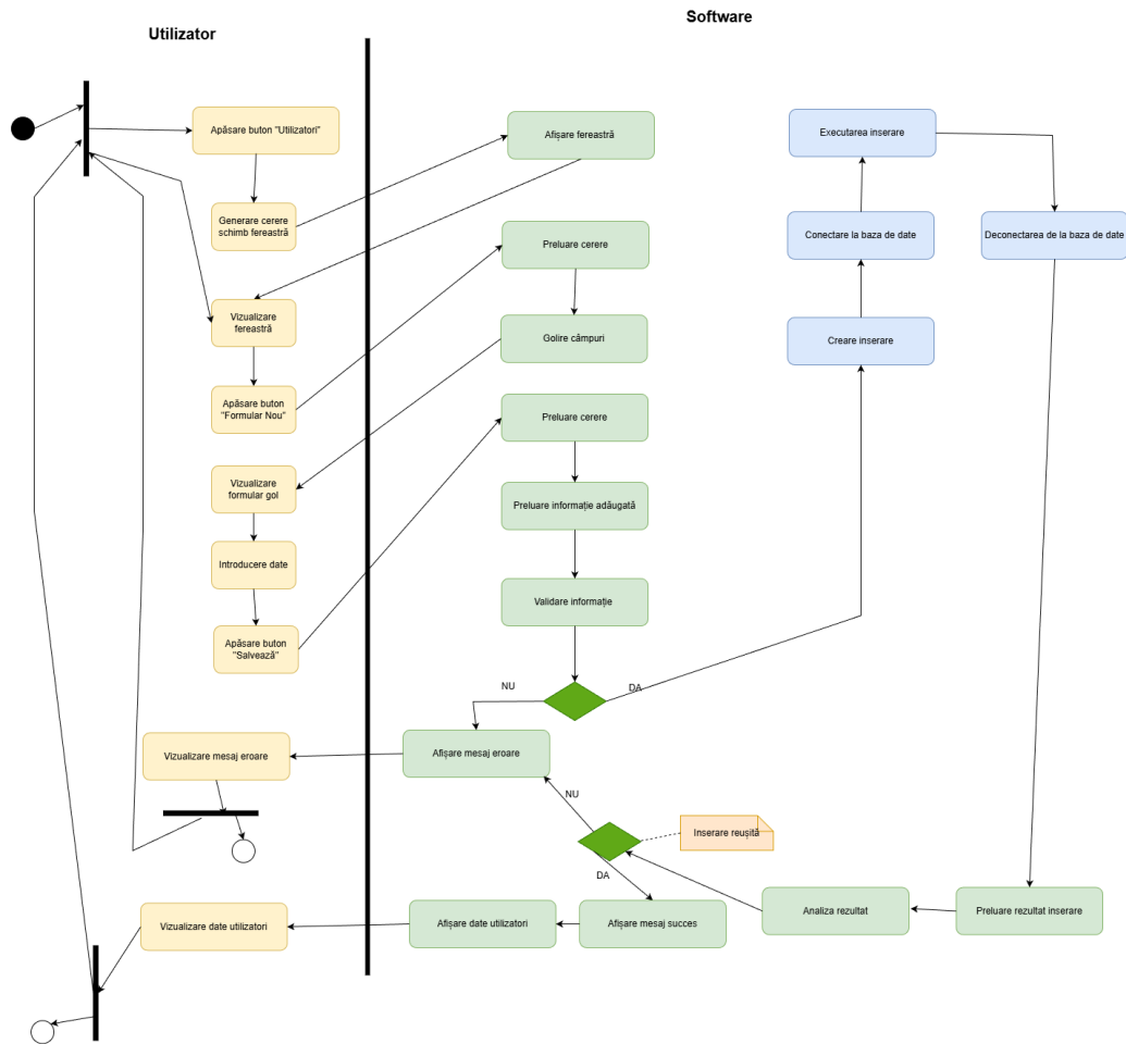
Figura 18: Diagrama de activități: Adăugare utilizator (Administrator)
