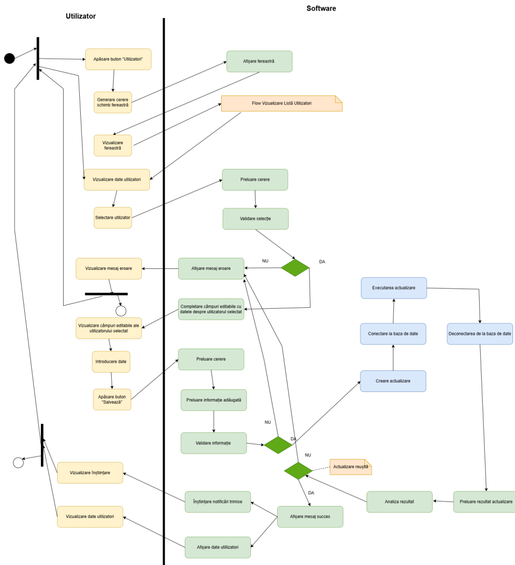
Figura 24: Diagrama de activități: Notificare și actualizare utilizator (Administrator)
