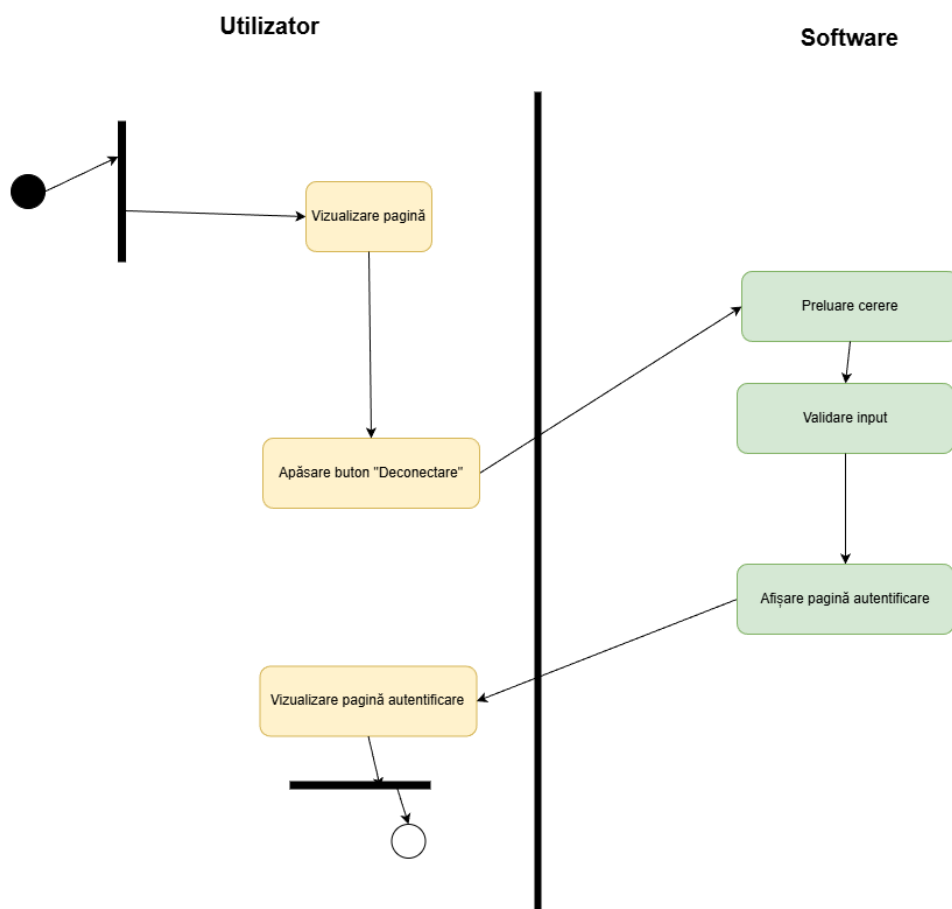
Figura 3: Diagrama de activități: Deconectare
