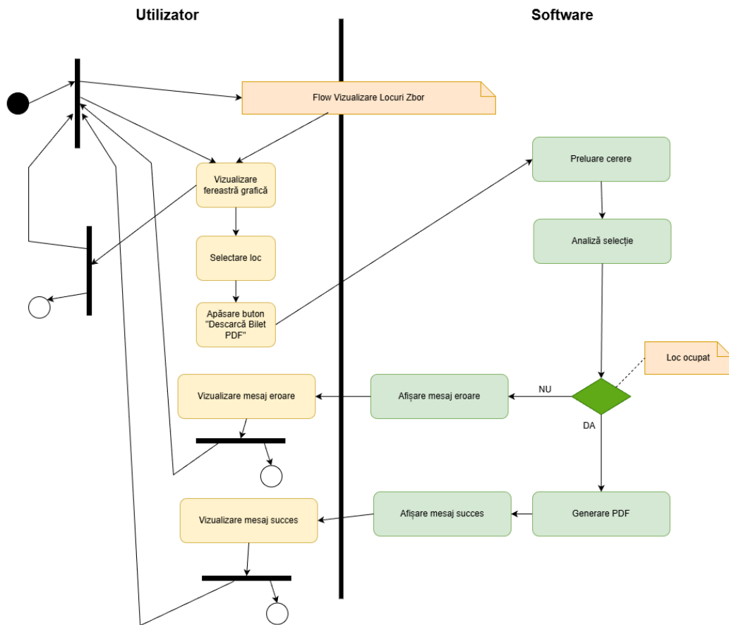
Figura 9: Diagrama de activități: Descărcare bilet PDF (Angajat)
