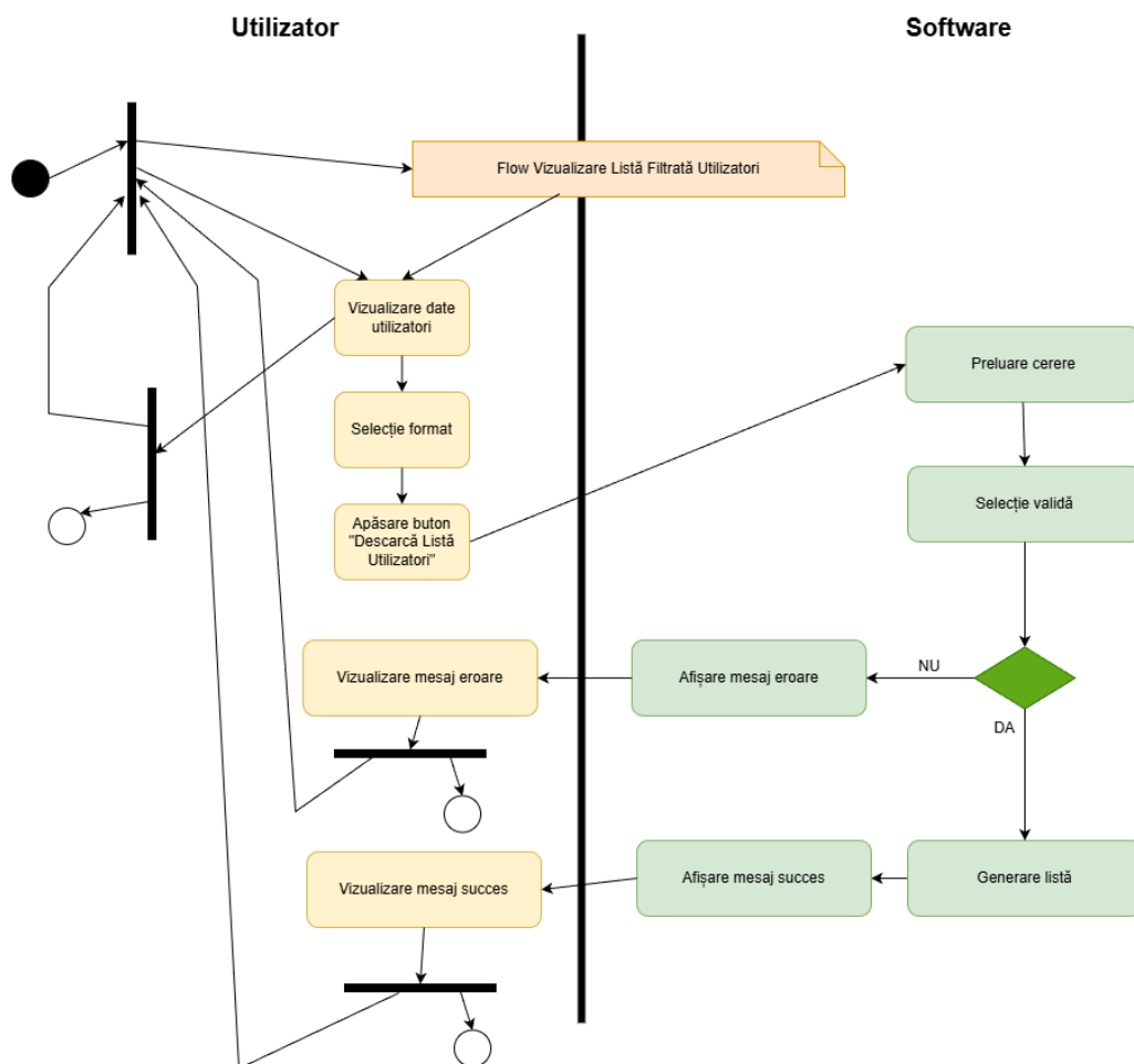
Figura 23: Diagrama de activități: Descărcare listă utilizatori (Administrator)
