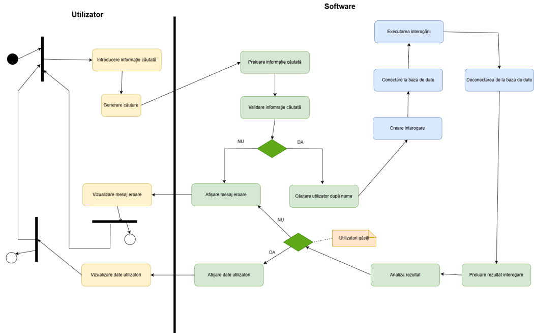
Figura 21: Diagrama de activități: Căutare utilizator (Administrator)
