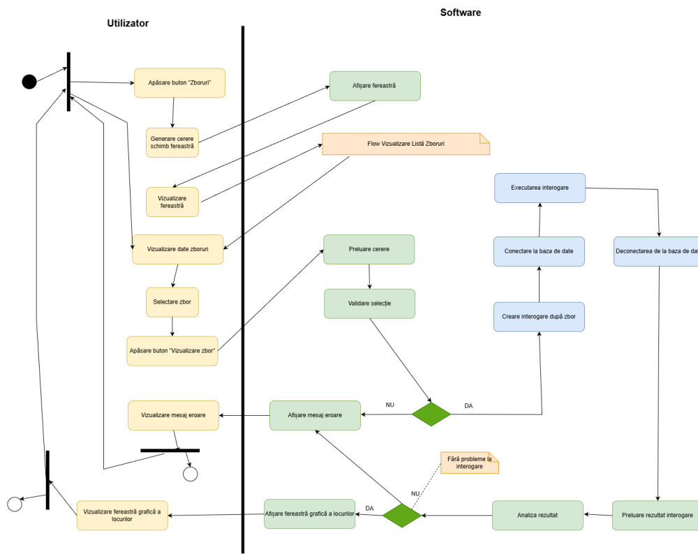
Figura 6: Diagrama de activități: Vizualizare grafică a locurilor (Angajat)
