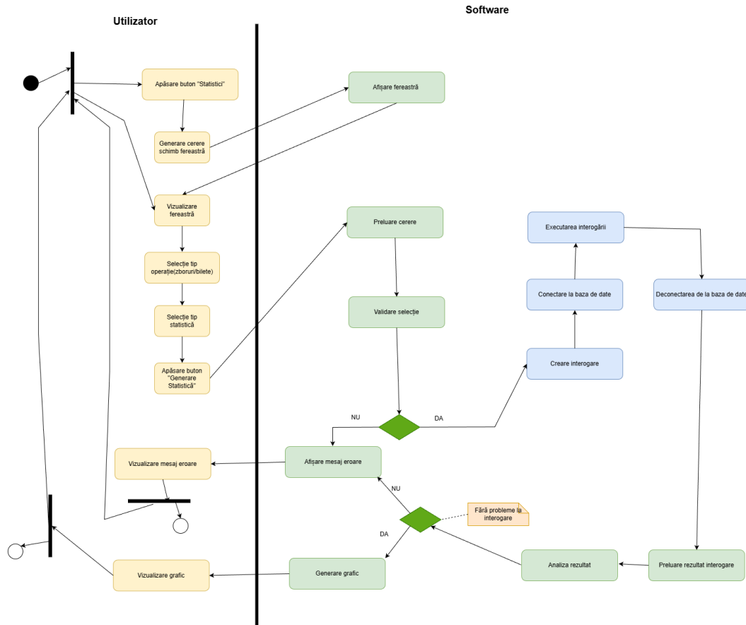
Figura 16: Diagrama de activități: Vizualizare statistică (Manager)
