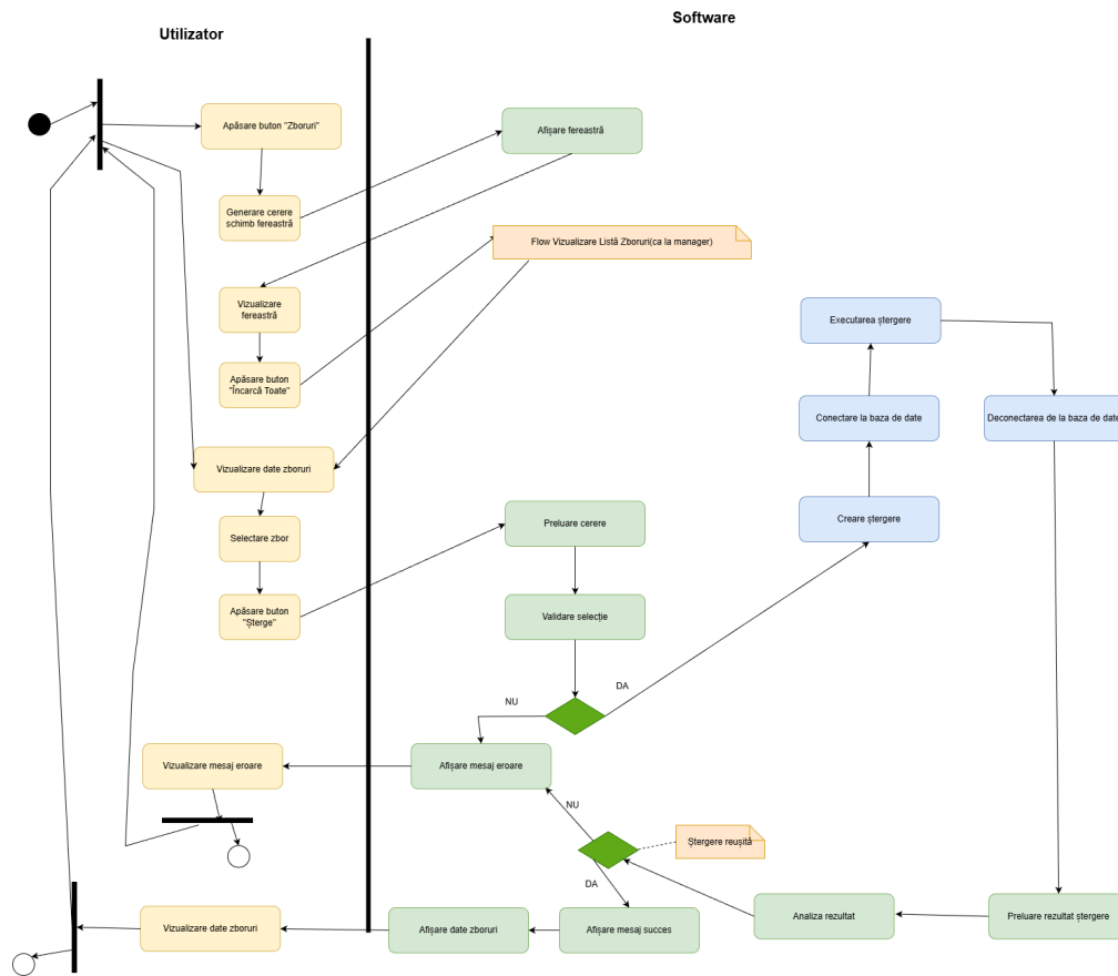
Figura 13: Diagrama de activități: Ștergere zbor (Manager)
