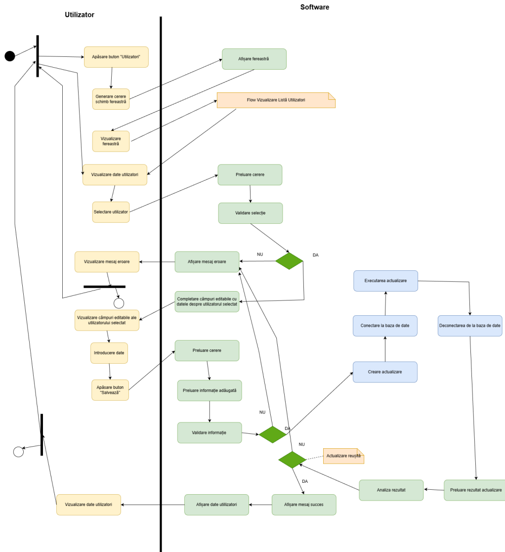
Figura 19: Diagrama de activități: Actualizare utilizator (Administrator)
