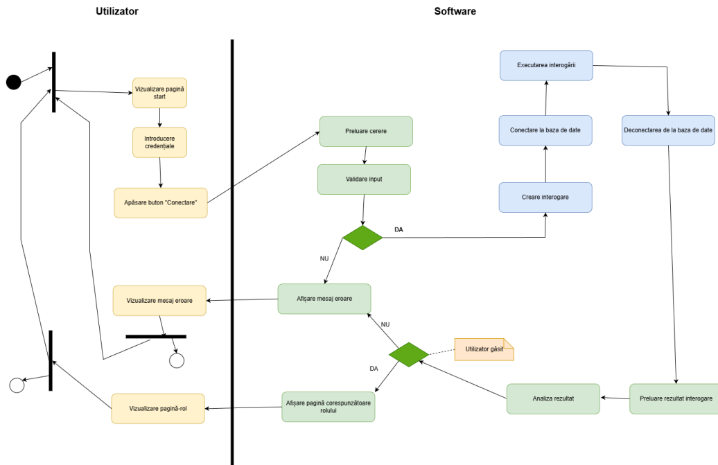
Figura 2: Diagrama de activități: Autentificare
