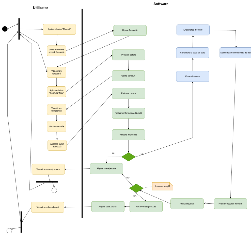
Figura 11: Diagrama de activități: Adăugare zbor (Manager)
