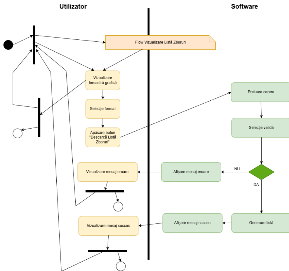
Figura 15: Diagrama de activități: Descărcare listă zboruri (Manager)
