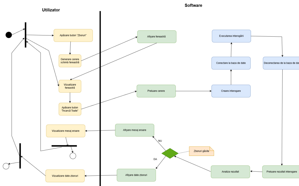
Figura 5: Diagrama de activități: Vizualizare listă zboruri (Angajat)
