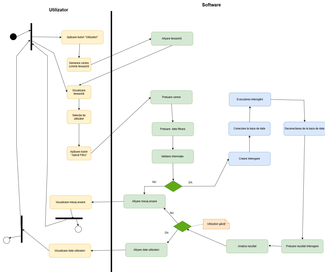
Figura 22: Diagrama de activități: Filtrare listă utilizatori (Administrator)
