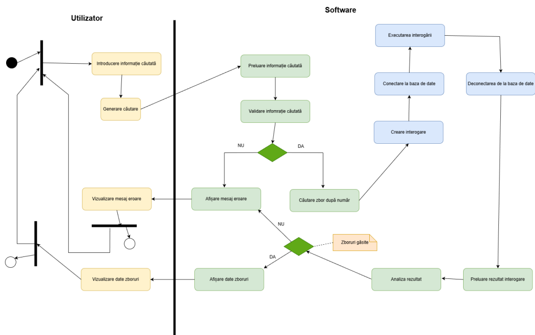
Figura 14: Diagrama de activități: Căutare zbor (Manager)
