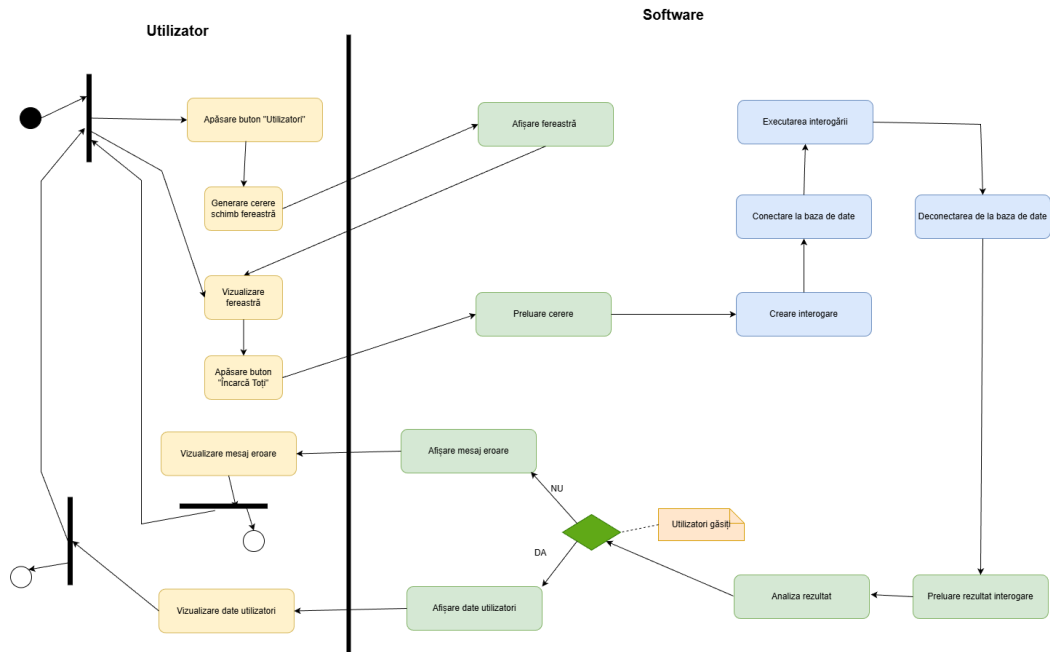
Figura 17: Diagrama de activități: Vizualizare listă utilizatori (Administrator)
