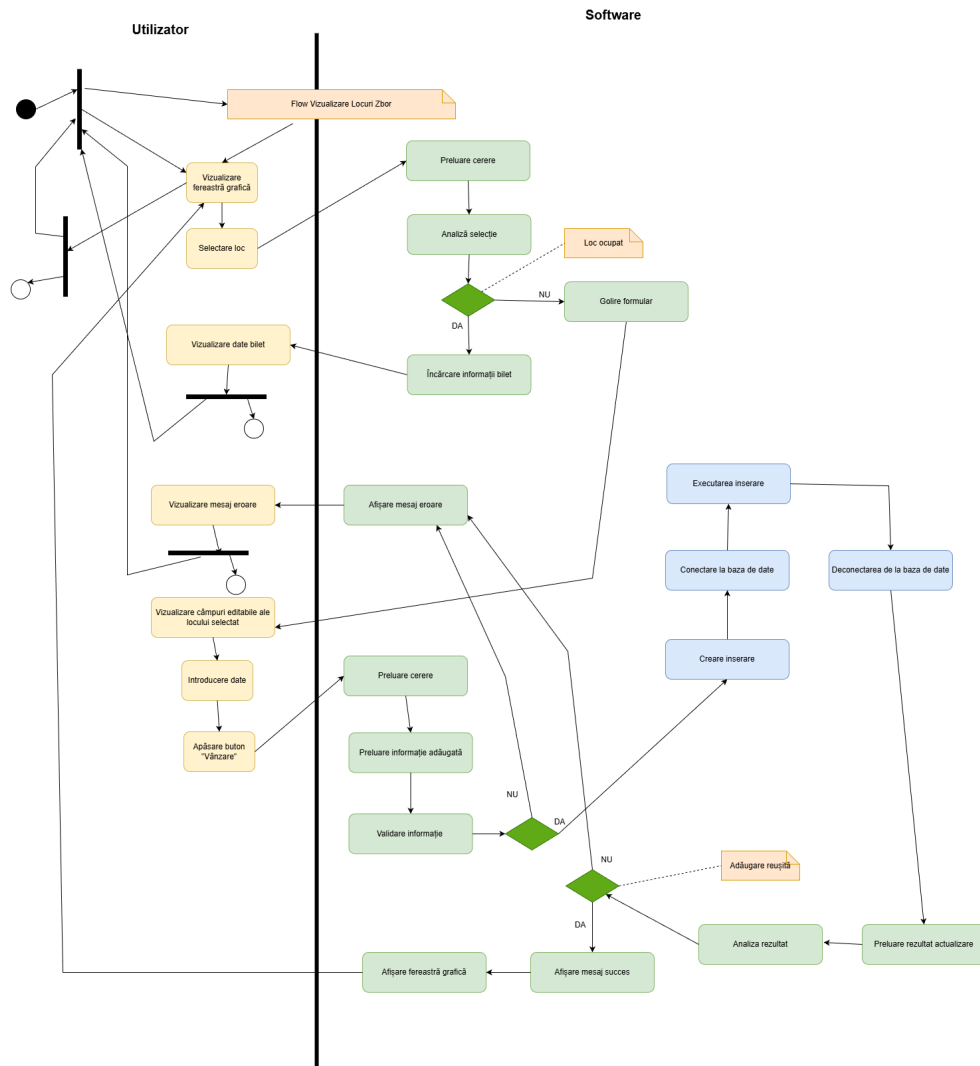
Figura 8: Diagrama de activități: Vânzare bilet (Angajat)
