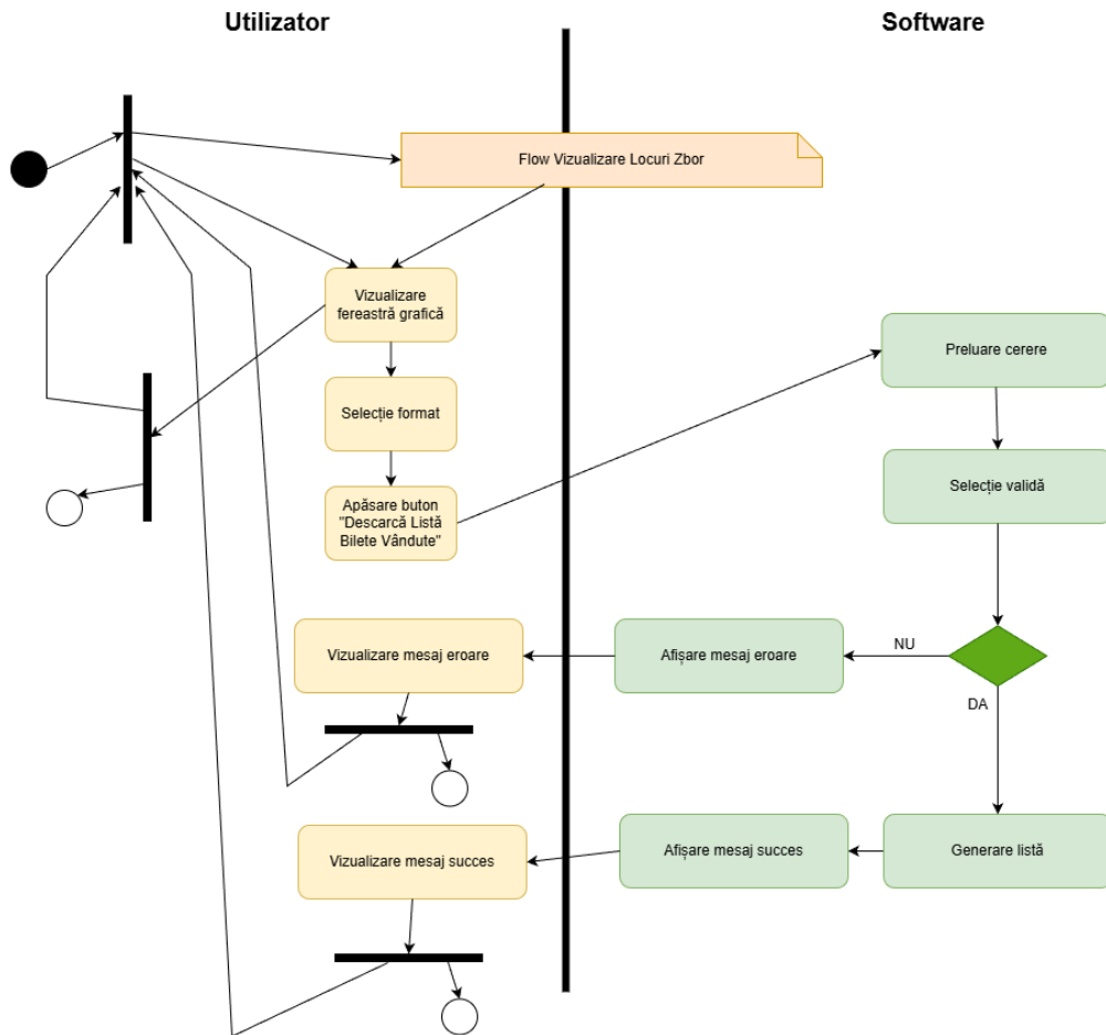
Figura 10: Diagrama de activități: Descărcare listă bilete vândute (Angajat)
