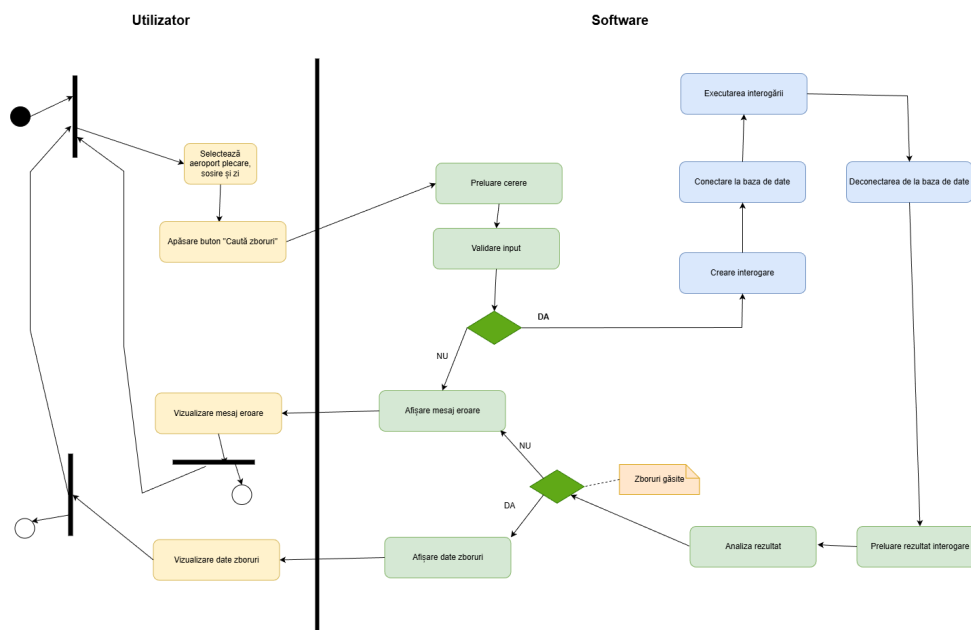
Figura 4: Diagrama de activități: Vizualizare zboruri dintre 2 aeroporturi
