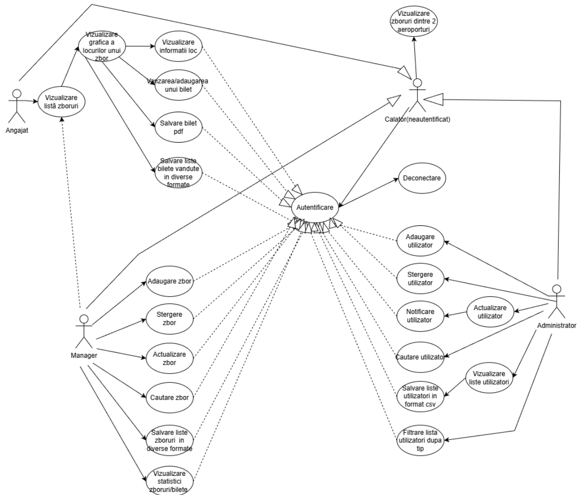
Figura 1: Diagrama cazurilor de utilizare
