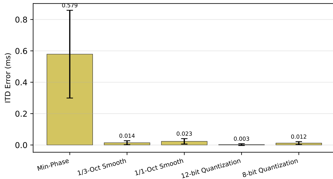
ITD Error (ms)
