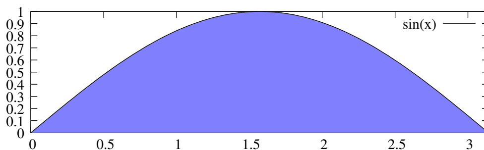
Obrázek 4.1: Výpočet integrálu metodou Monte Carlo
